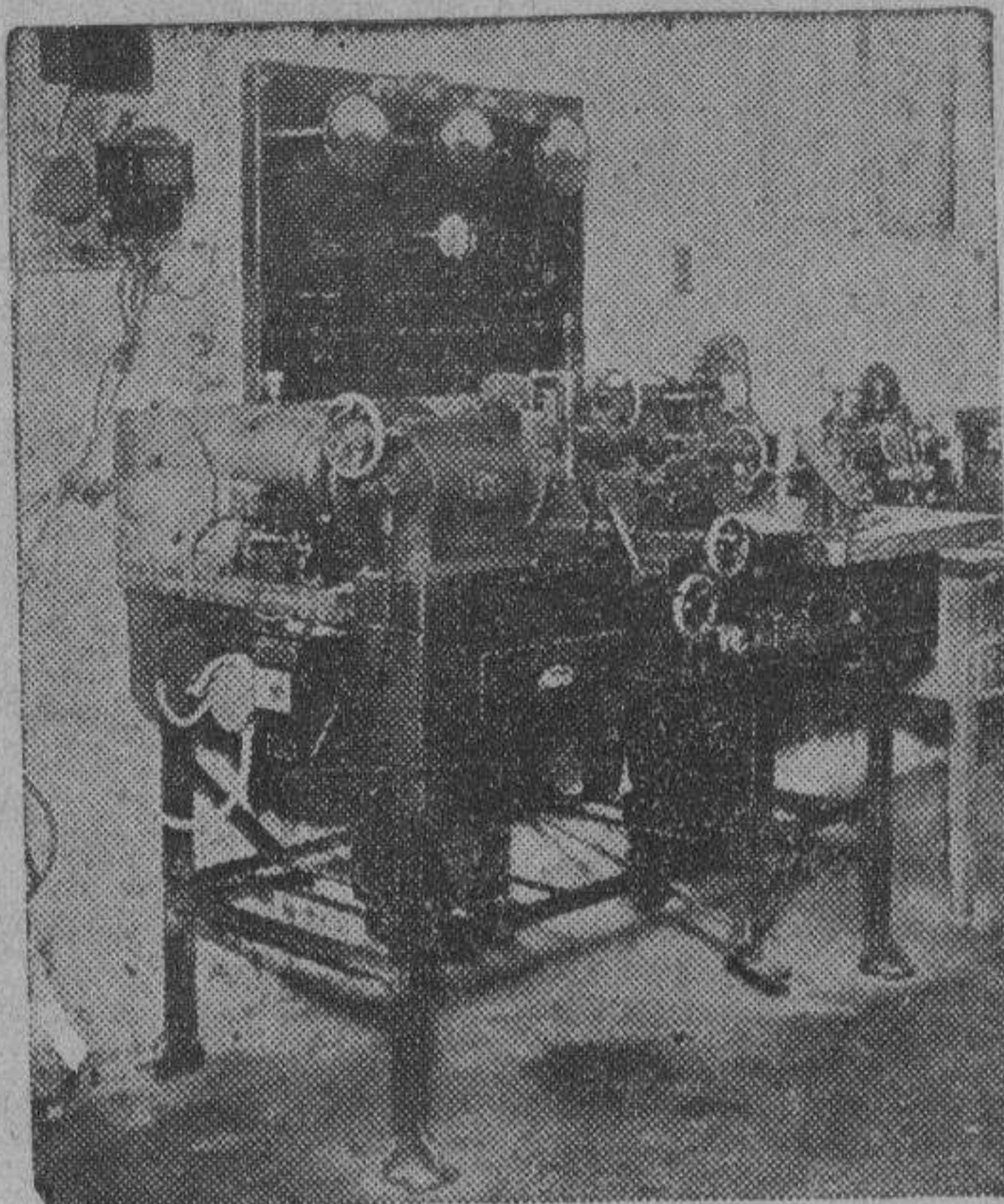
COMPROBADOR ELECTRICO RECIENTE INSTALADO para probar Condensadores, Bobinas, Generadores, Disparadores, Otros Aparatos Electricos y Velocímetros.
