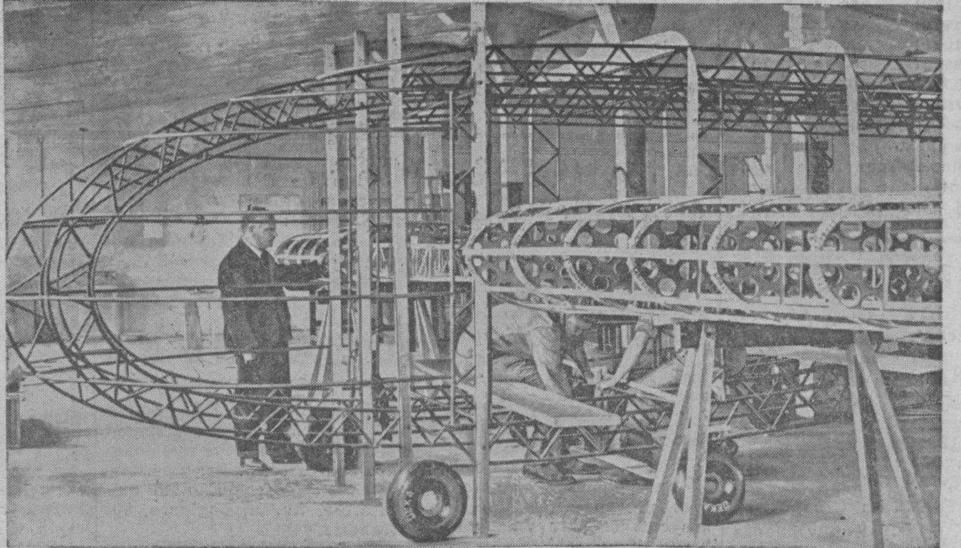
Presentamos el esqueleto de la maravillosa máquina de que hablamos hace pocos días. Es el helicóptero que, con los planos del ingeniero austriaco Wimputz, construye una gran fábrica inglesa. Afirman los técnicos que está resuelto el ascenso vertical y el descenso como con paracaídas.
