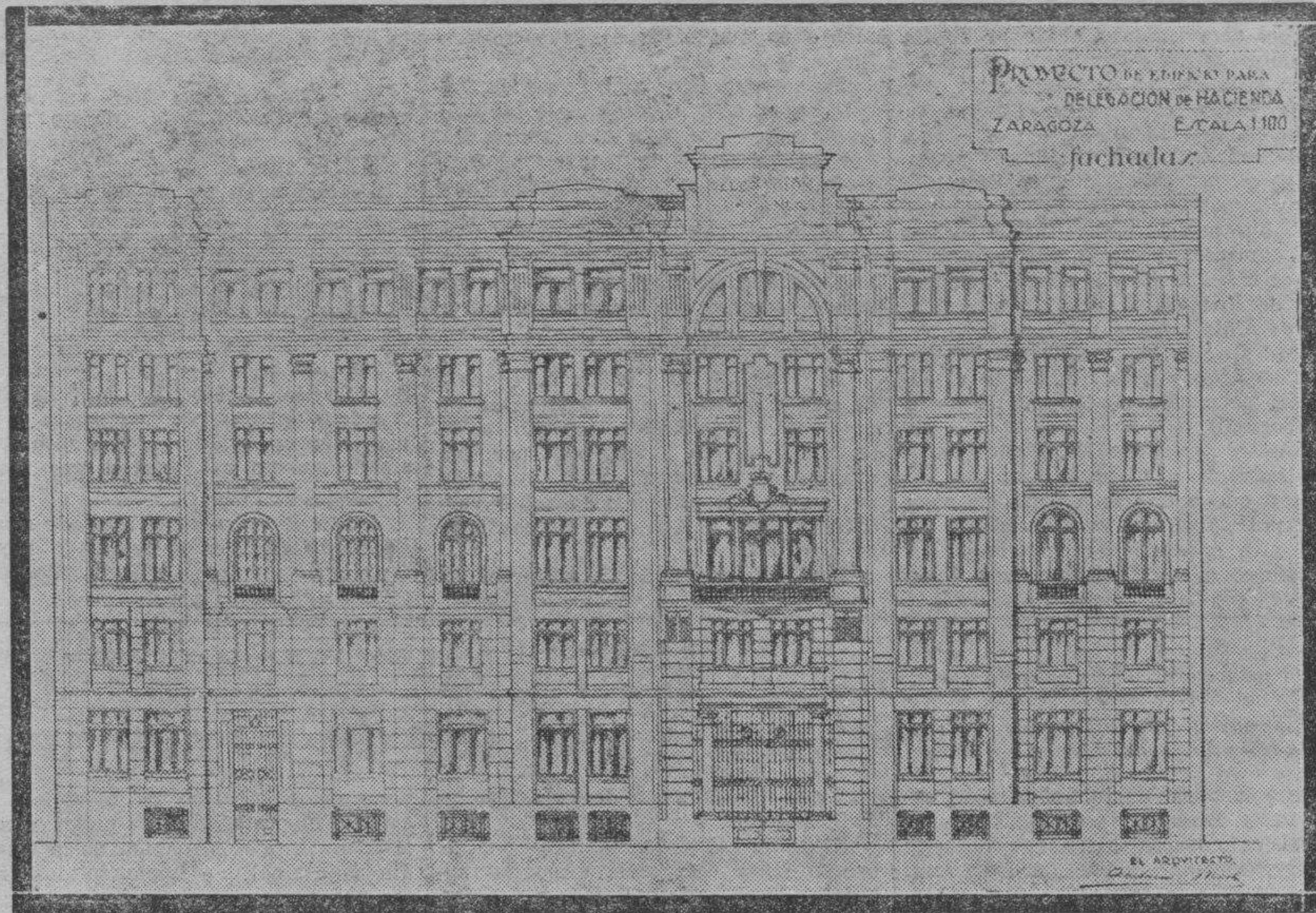
Proyecto del edificio para Delegación de Hacienda en Zaragoza, según el arquitecto señor Merlo.
