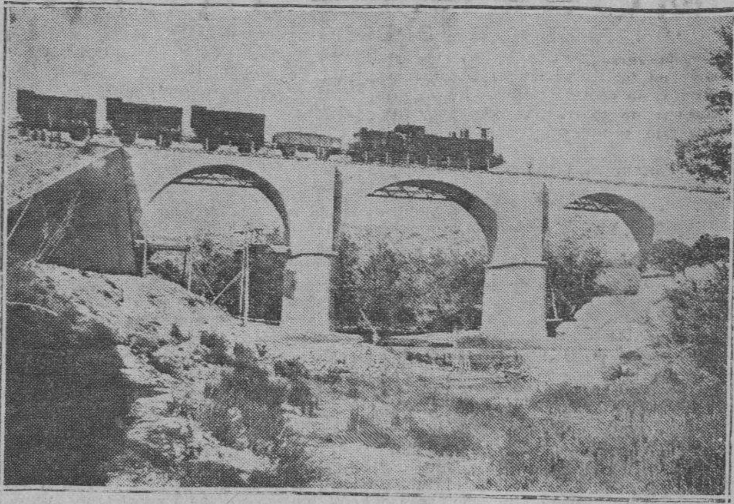
ALCANIZ.—Puenete sobre el río Martín, del ferrocarril de Val de Zafán a San Carlos, que, en virtud del tráfico que ha de desarrollarse en dicha línea, ha precisado efectuarse la reforma de ensanche y reforzamiento
