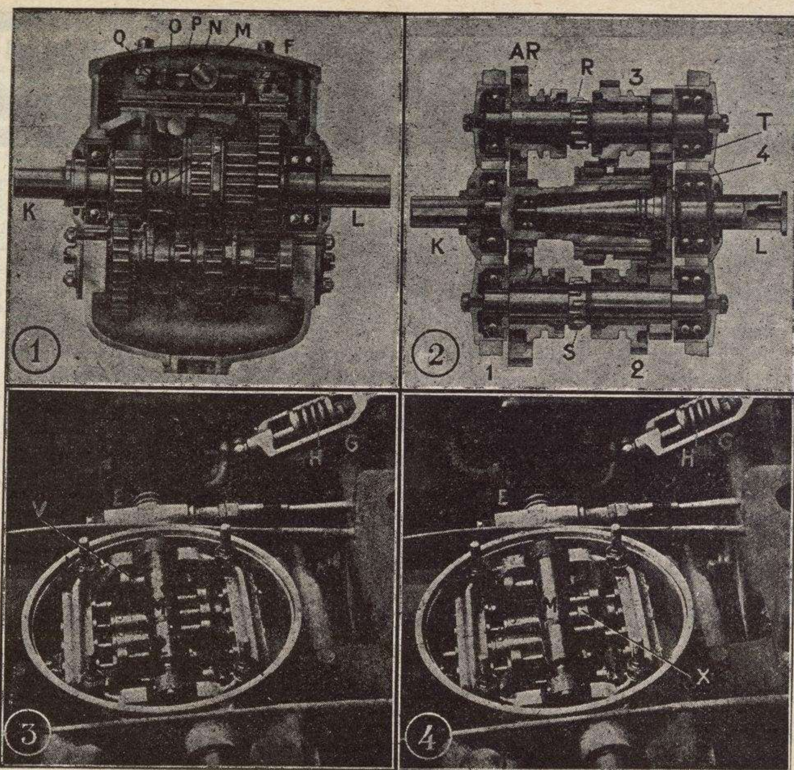
Detalles de la caja de velocidades ZF
