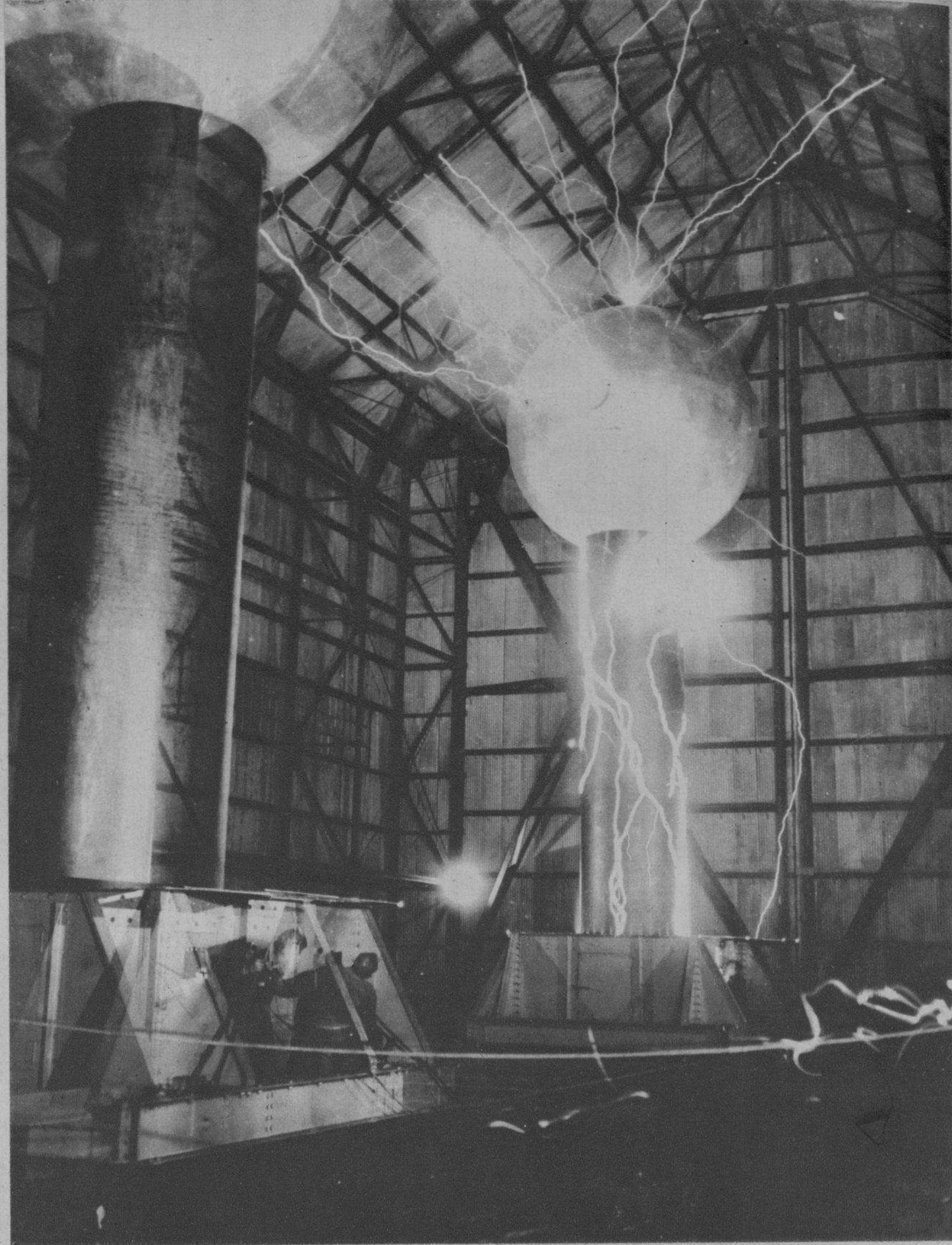
RAYO ELECTRICO PODEROSISIMO. En Round Hill, Estado de Massachusetts, fué hecha esta prueba de producir un rayo por medio de una corriente eléctrica de siete millones de voltios. El hombre, en su afán de superarse, llega a tener el mismo poder de la naturaleza. Dicen los que vieron la prueba que esta lámpara de Aladino iluminará muchos puntos oscuros de la ciencia (Foto Wide World)
