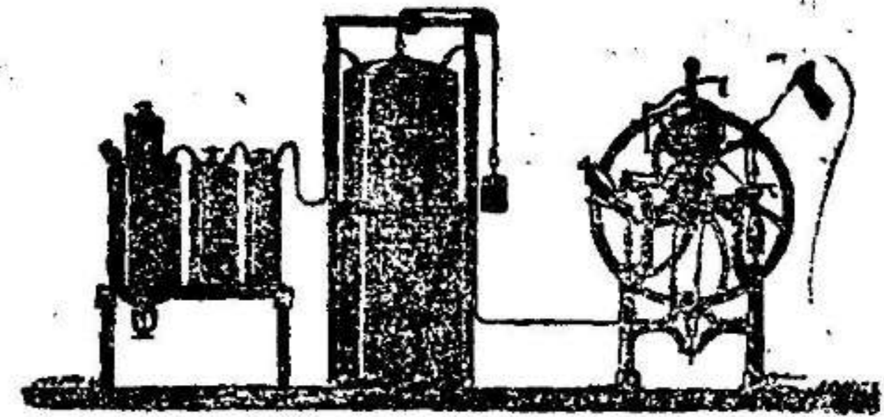
Aparatos para gaseosas, continuo, con embotelladoras unidas.
