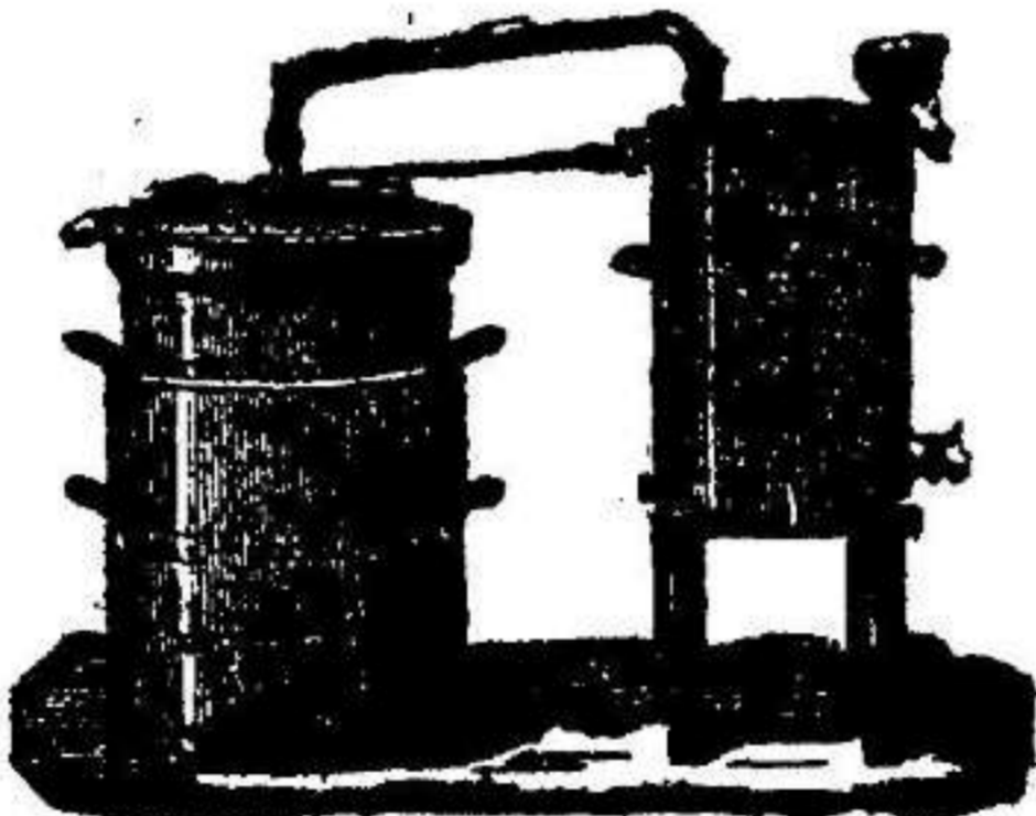
Alambique.
