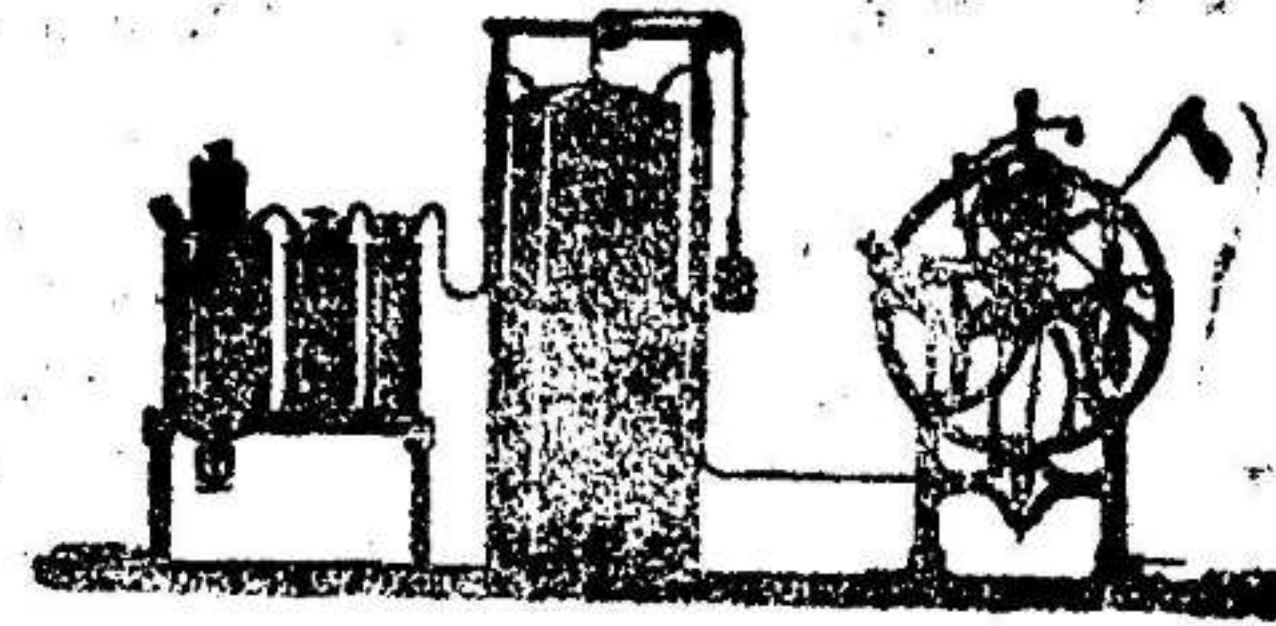
Aparato para gaseosas, continuo, con embotelladoras unidas.
