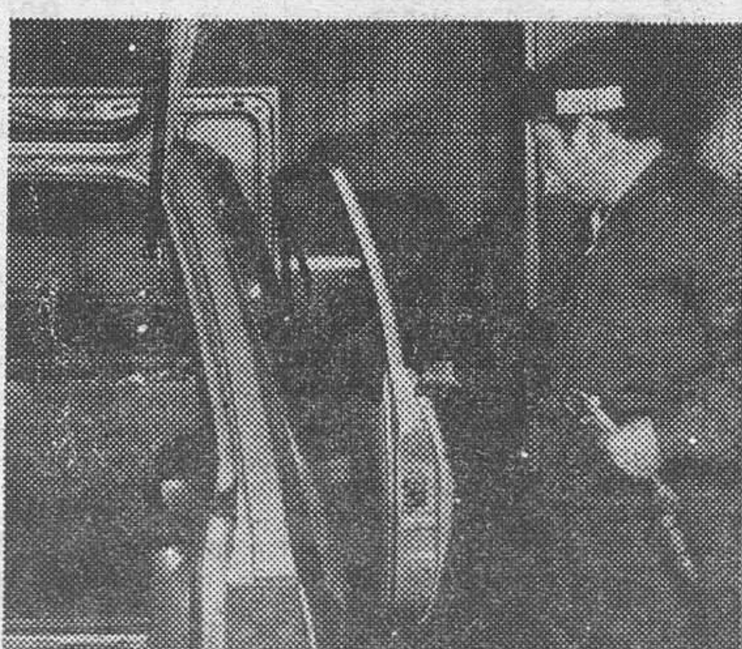
Inyección del DINITROL ML en la puerta
