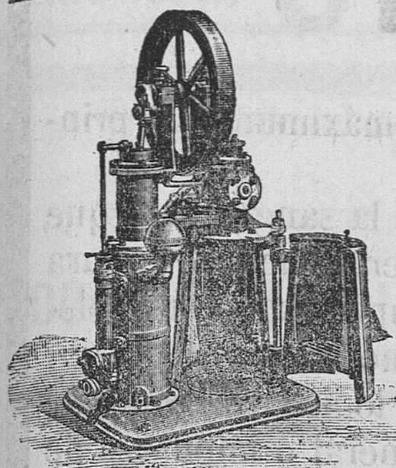
Motor con el hogar abierto para su inspección.
