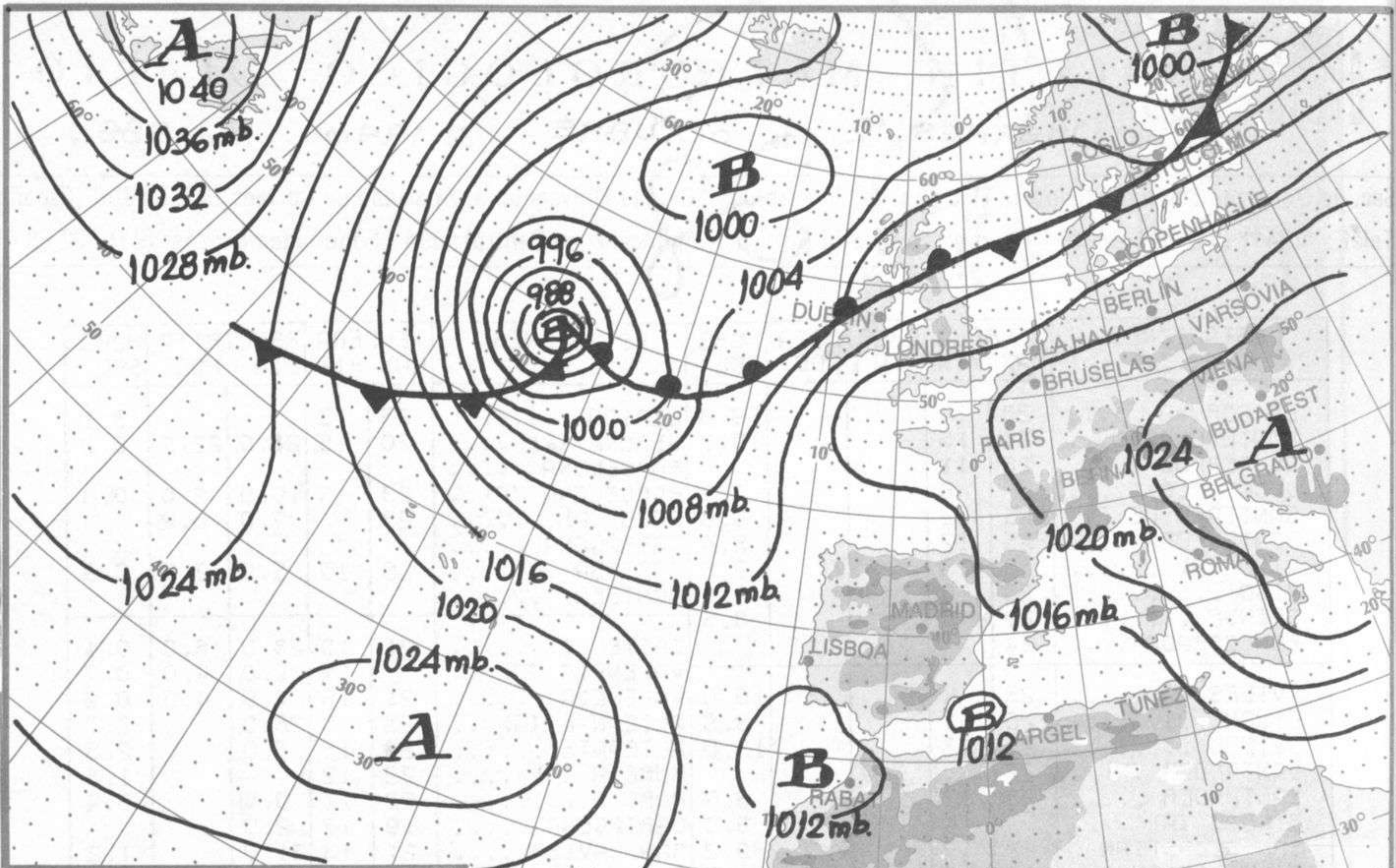
ANALISIS EN SUPERFICIE a 12 h. (TMG) Día 11-10-90
