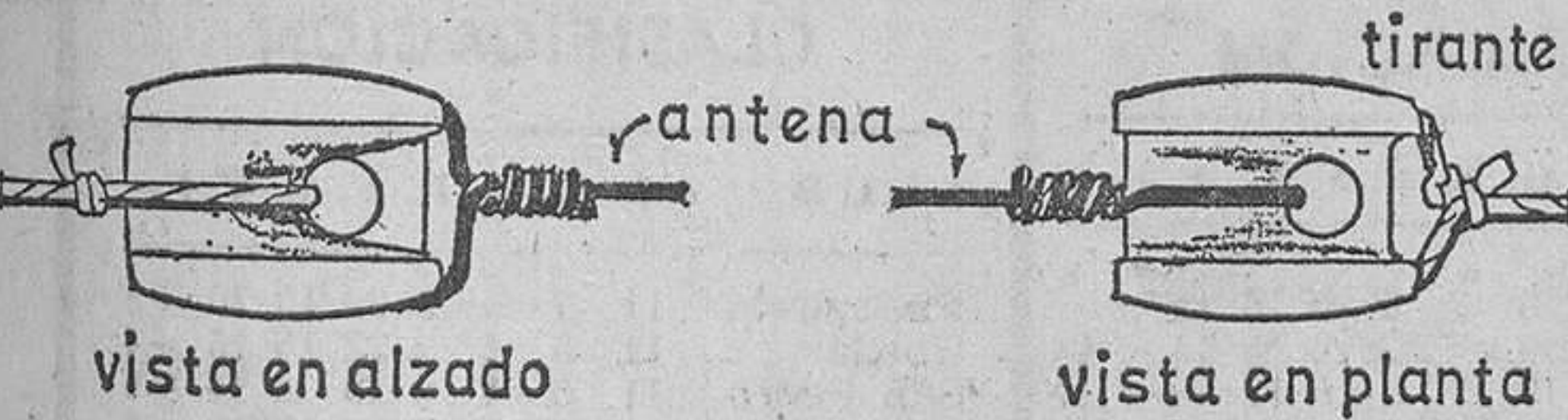
DETALLE DEL AISLADOR
