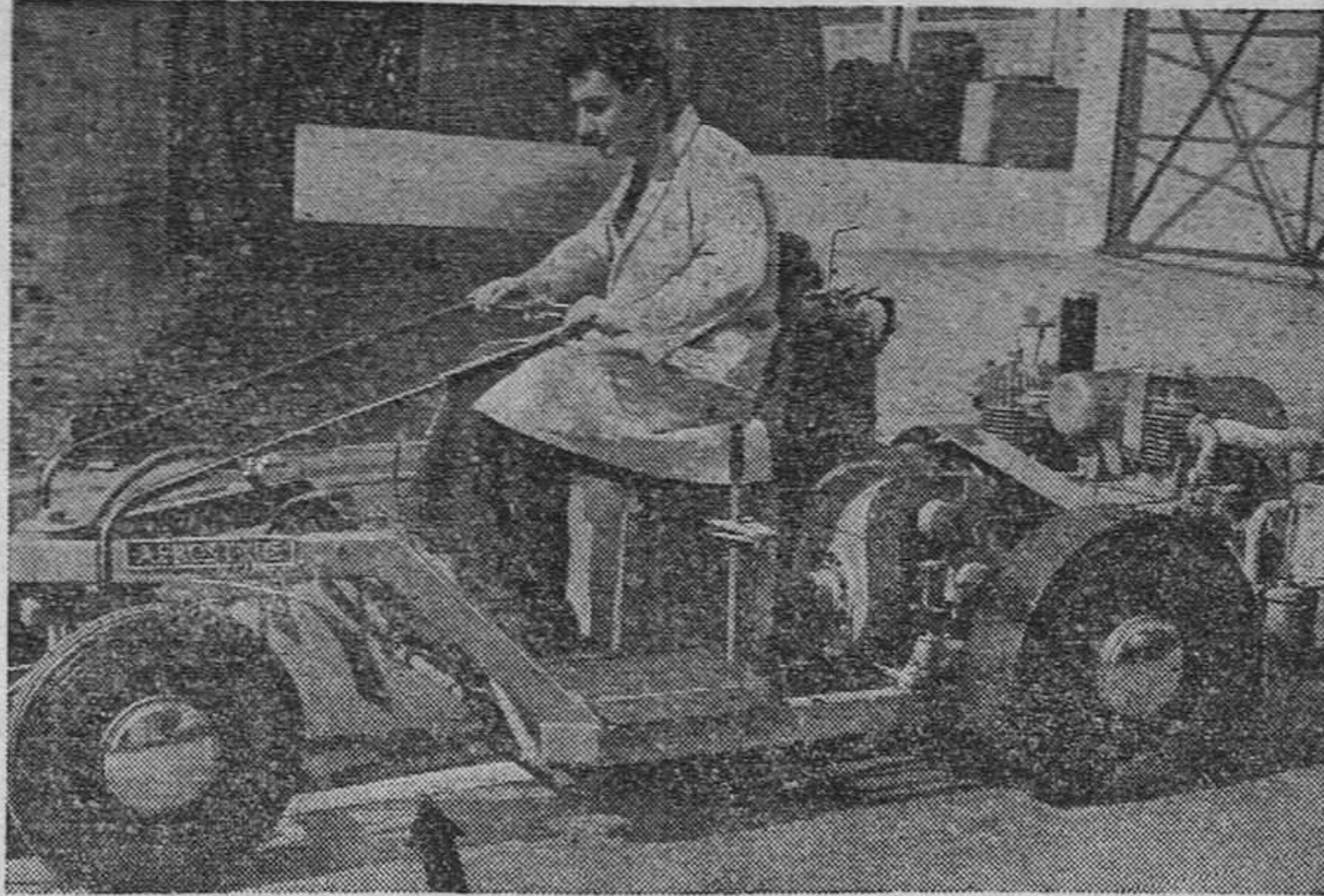
LONDRES.—La nueva máquina de marcar carreteras Aerostyle, que ha entrado en servicio para trazar líneas blancas a una velocidad de 35 kilómetros por día. Con esta máquina se emplea un nuevo tipo de pintura plástica y las líneas tienen una gran permanencia.—(Foto Calpe.)
