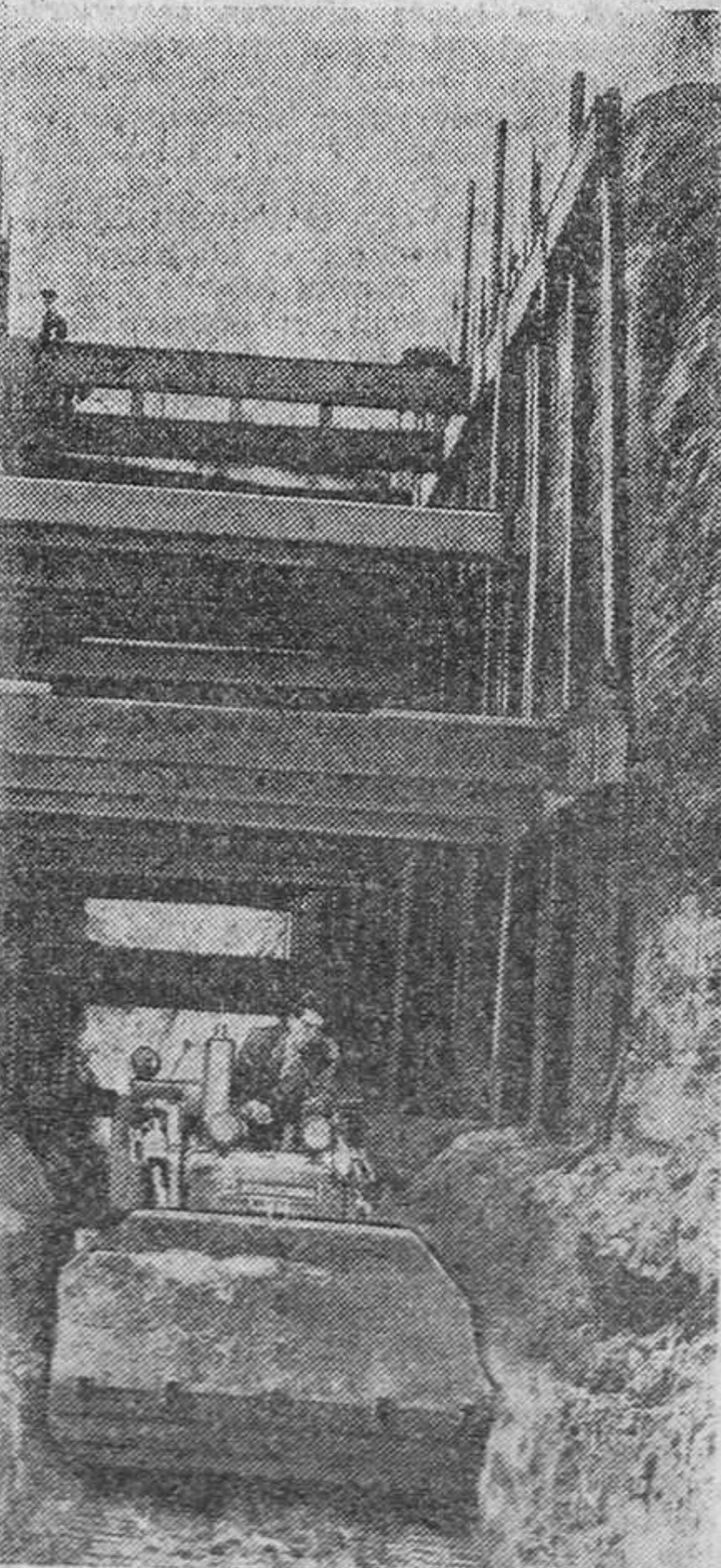
Esta máquina está cortando, con toda precisión, un monte, para permitir la colocación de un puente para una nueva carretera de circunvalación en Farnham (Inglaterra). Comenzando en la parte más alta del monte, la máquina trabajó en secciones de 60 centímetros de profundidad, transportó la tierra y la cargó en camiones. Sin otro equipo auxiliar para esta labor, el corte entero, hasta el nivel necesario, que fué de 1.146 metros cúbicos, se verificó en pocos días de labor. — (Foto Calpe).
