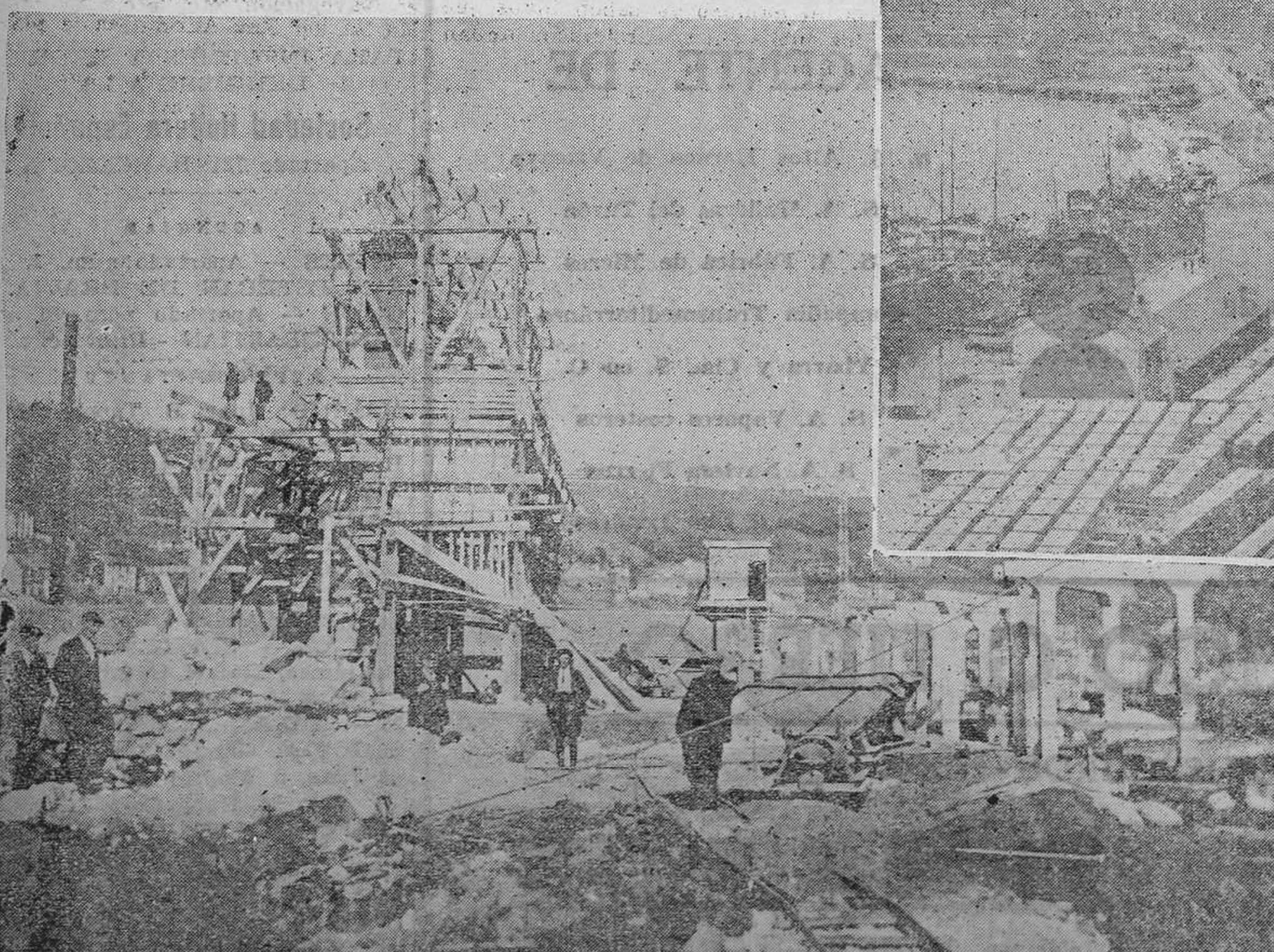
SAN ESTEBAN DE PRAVIA.—Construcción de los nuevos cargaderos que darán el máximo rendimiento al embarque de carbón y que irá emplazado en el dique oeste, cuyas obras se ejecutan actualmente (Foto archivo REGION.)
