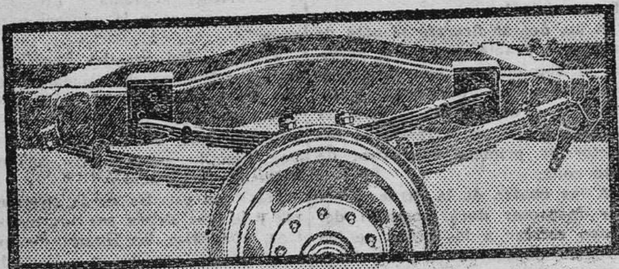
Las ballestas auxiliares traseras aseguran una mejor suspensión de la carga y una mayor estabilidad del camión.
