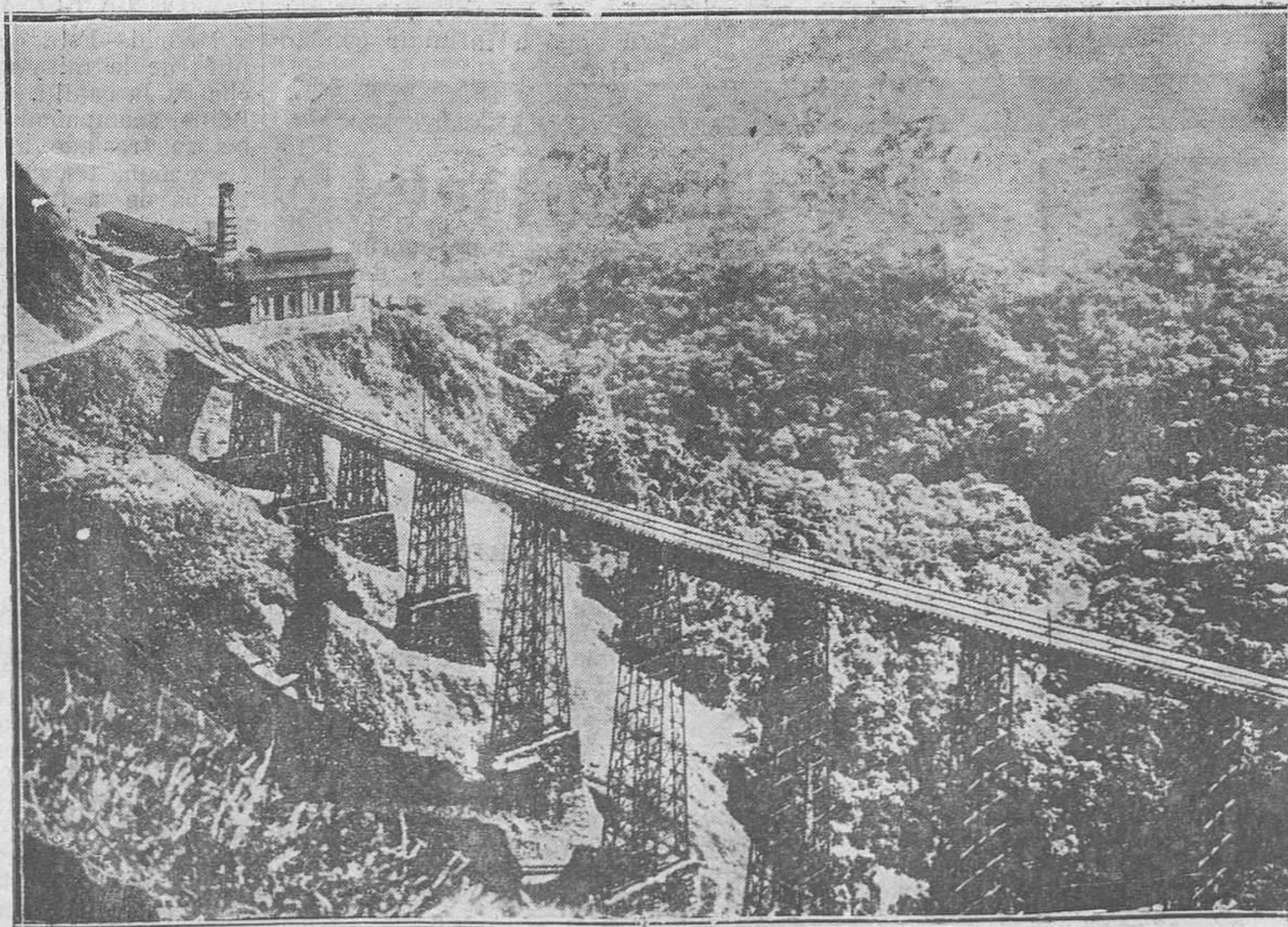
UNA OBRA MAESTRA DE INGENIERIA.—El trozo de ferrocarril más peligroso del mundo.—La unión entre San Paolo y Santos (Brasil).—Ingenieros alemanes han dirigido la construcción.—El viaducto, en algunos trozos, tiene más de 200 metros de altura (Foto VIDAL)
