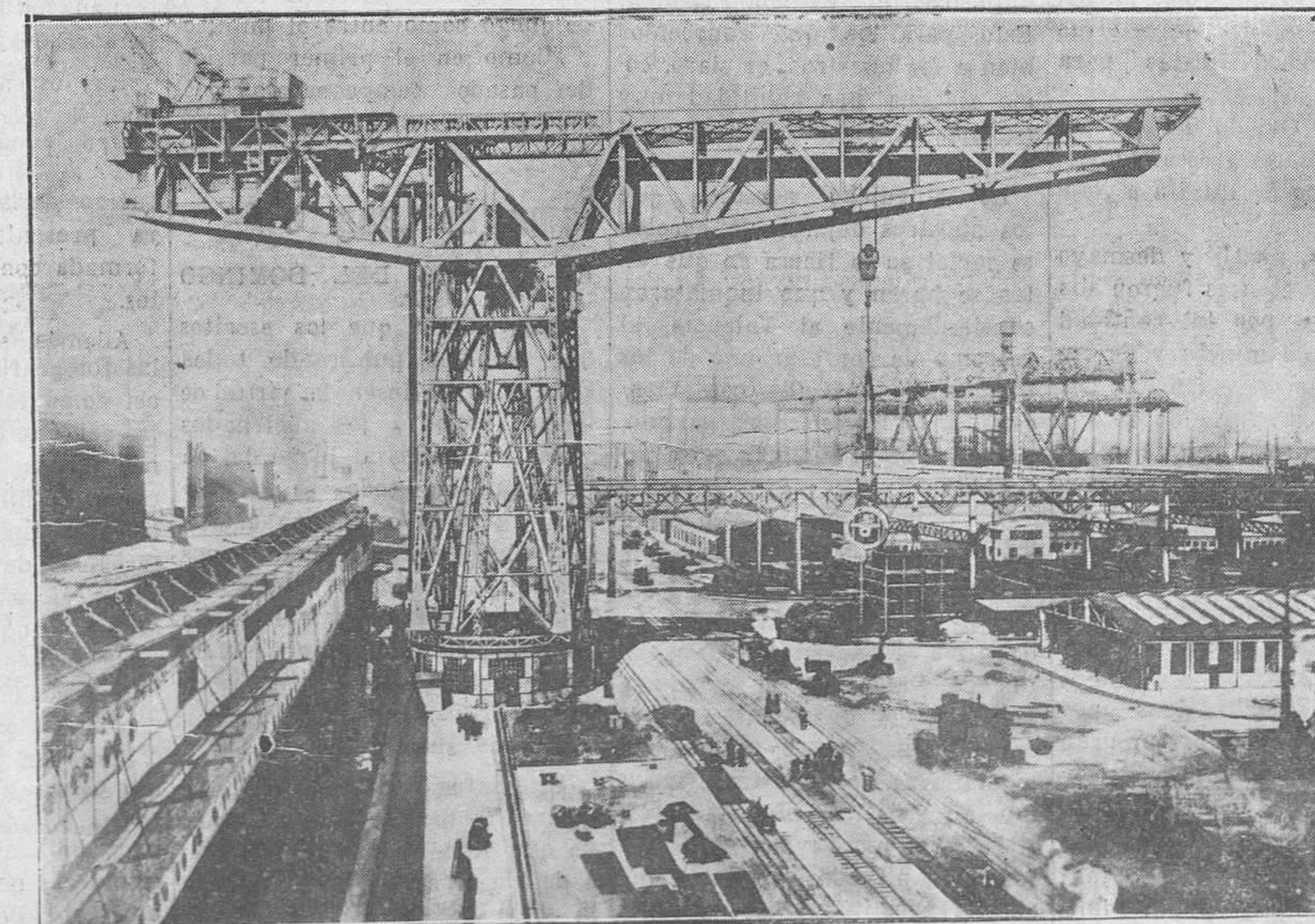
EL TRIUNFO DE LA TECNICA.—La sociedad Demag, de Duisburg, ha construido para el muelle de Hamburgo una gigantesca grúa, cuyos brazos, en posición elevada, alcanzan la altura de la catedral de Múnic. (VIDAL)
