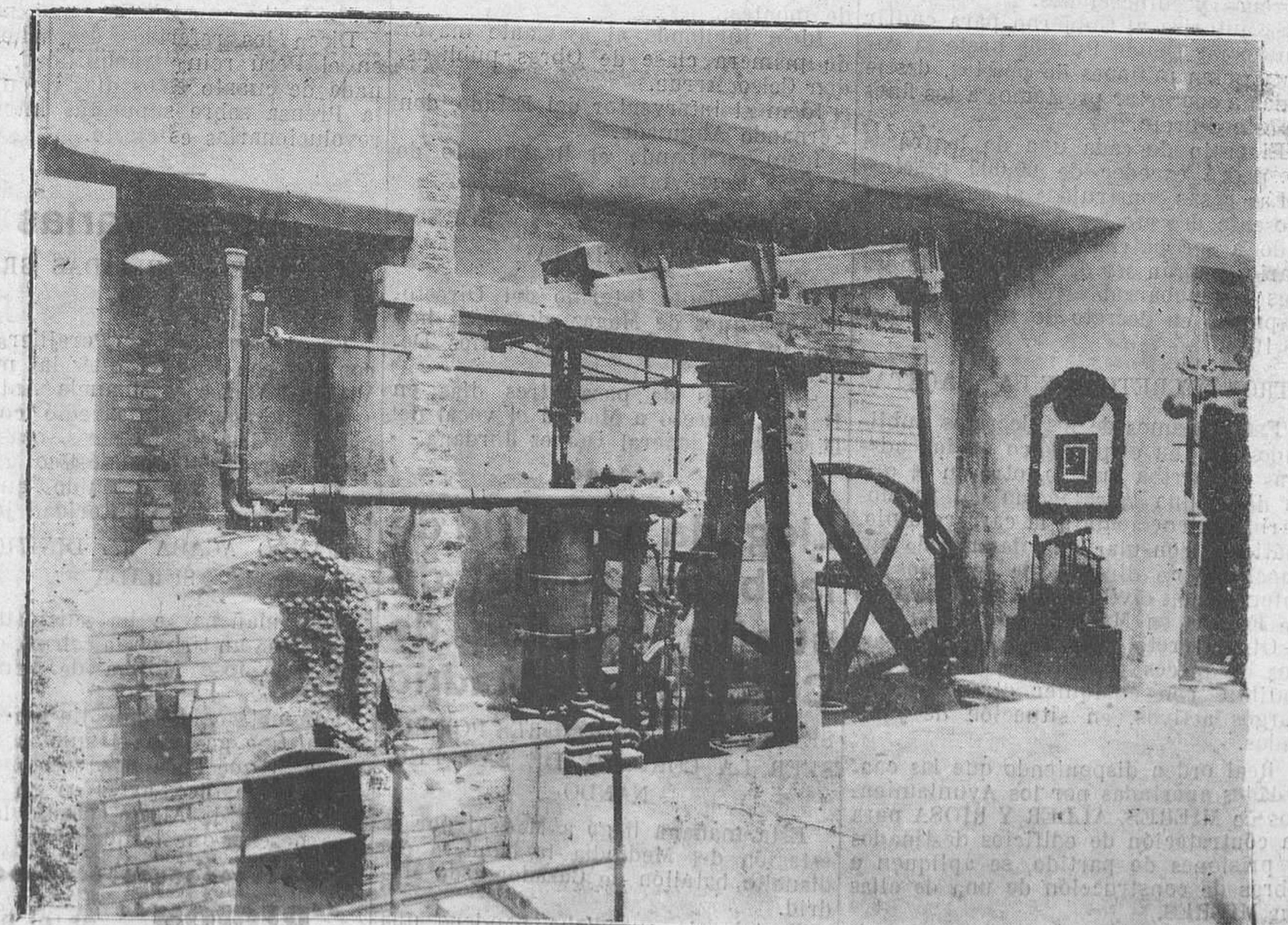
DEL MUSEO ALEMÁN DE MUNICH.-Máquina Watt, del año 1788, con caldera en forma de baul.
