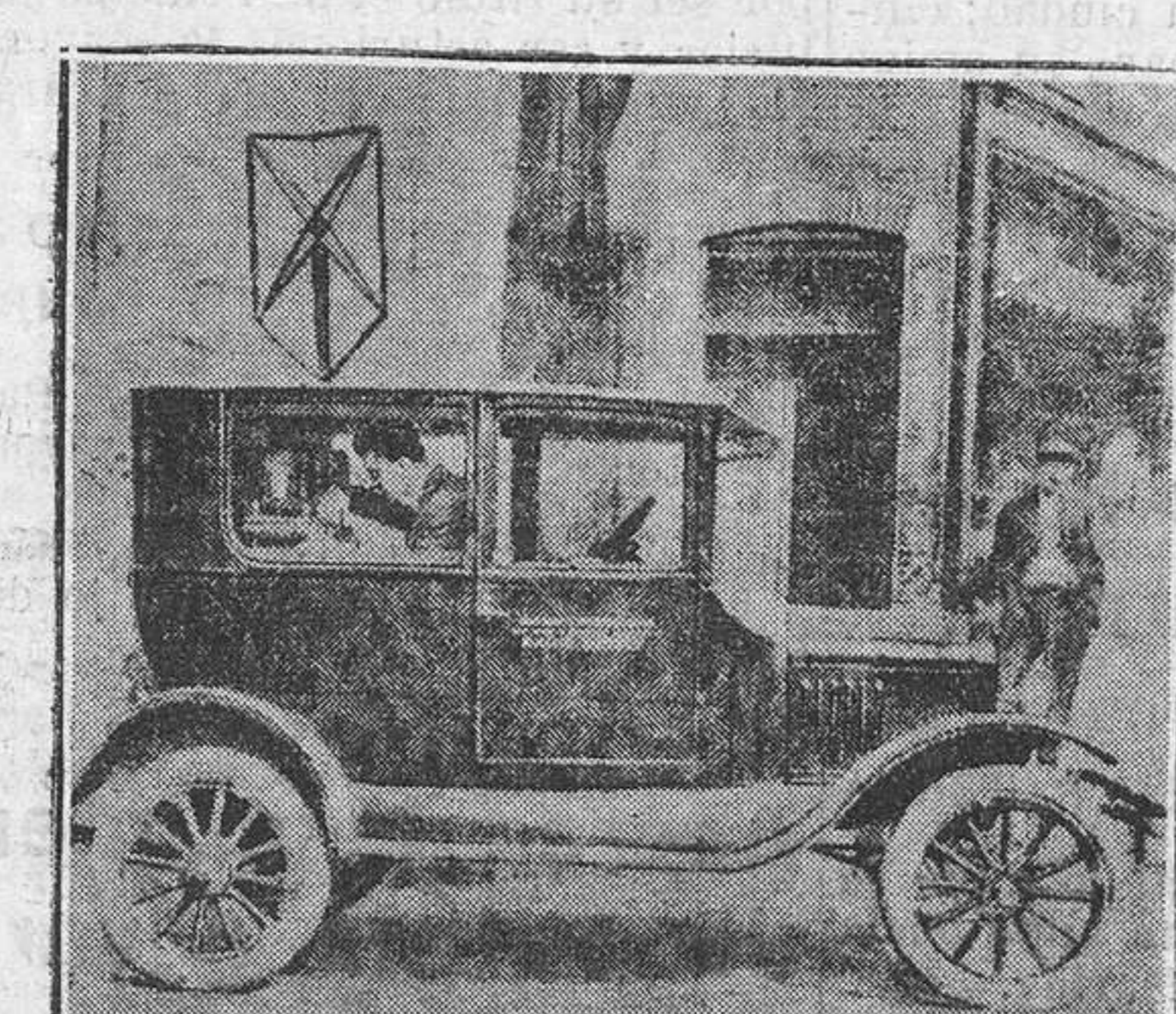
Uno de los automóviles de que dispone la Universidad americana de Pennsylvania, provisto de una completísima instalación radiotelefónica para el estudio de las ondas de propagación.
