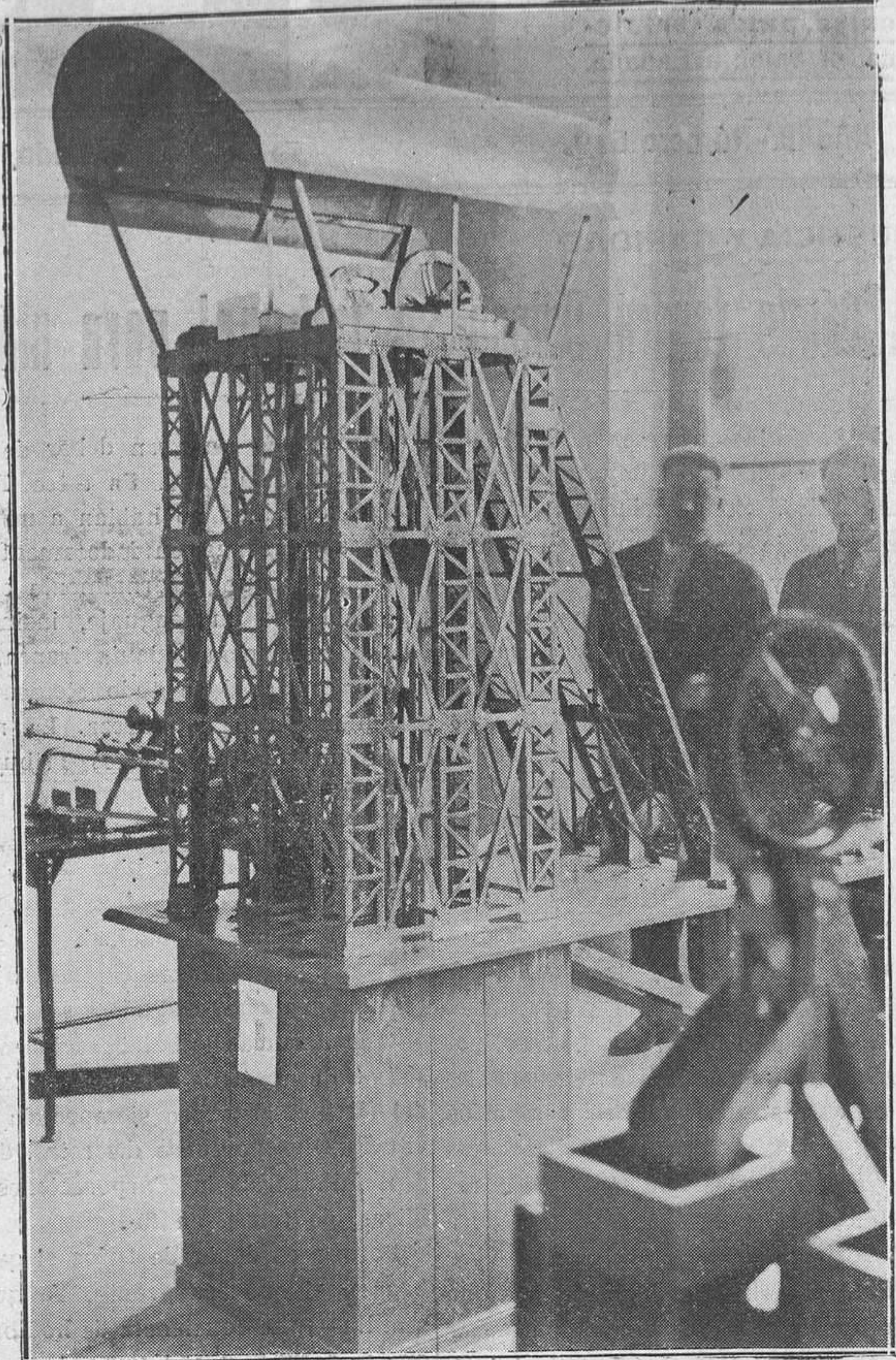
LA FELGUERA: DEL CERTAMEN DEL TRABAJO.-Castillete en miniatura del que existe en el pozo de "Peña-Rubia", con un paracaídas, inventado por los obreros Dimas Coalla y Manuel Blanco, autores a la vez de esta obra. (Foto M. Abad)
