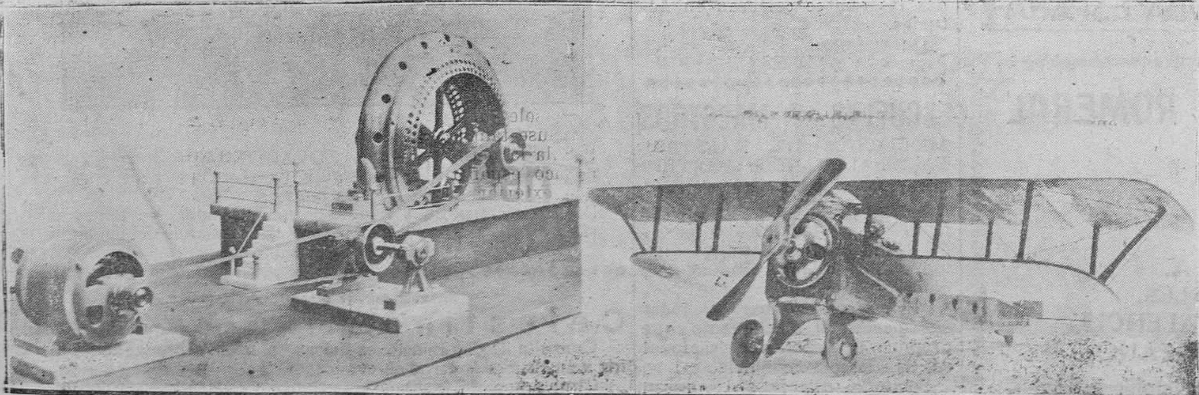
La Felguera.-Alternador trifasico de 24 polos, expuesto en el Certamen Provincial del Trabajo, por Nicomedes Santos de Avilés
