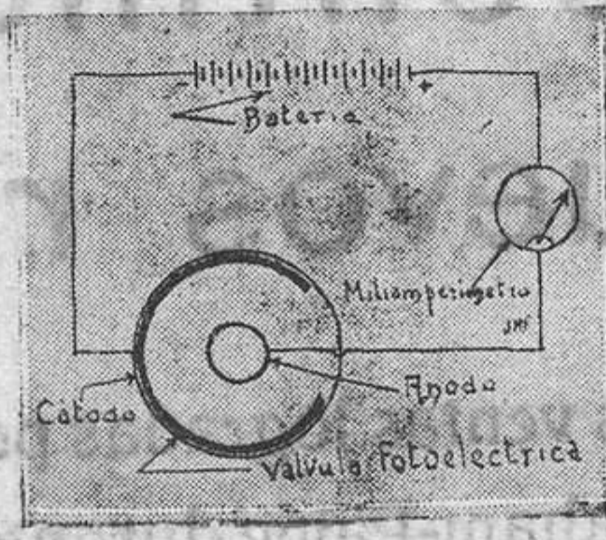
Esquema de la válvula fotoeléctrica
