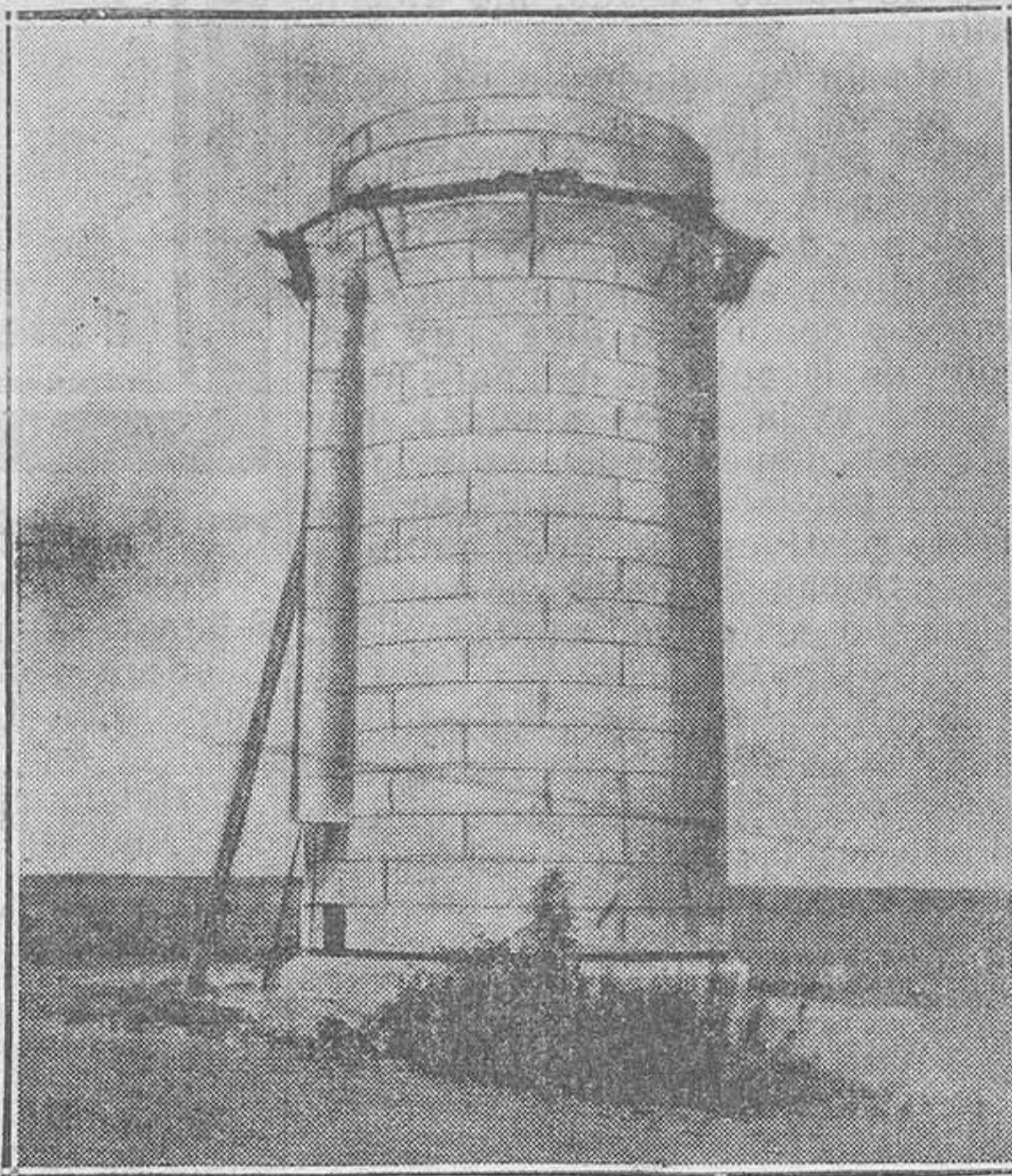
SILO VERTICAL EN CURSO DE MONTAJE.--Gracias a los aparatos móviles que se colocan a voluntad a más o menos altura, no es necesario elevar costoso andamiaje para montarlo.
