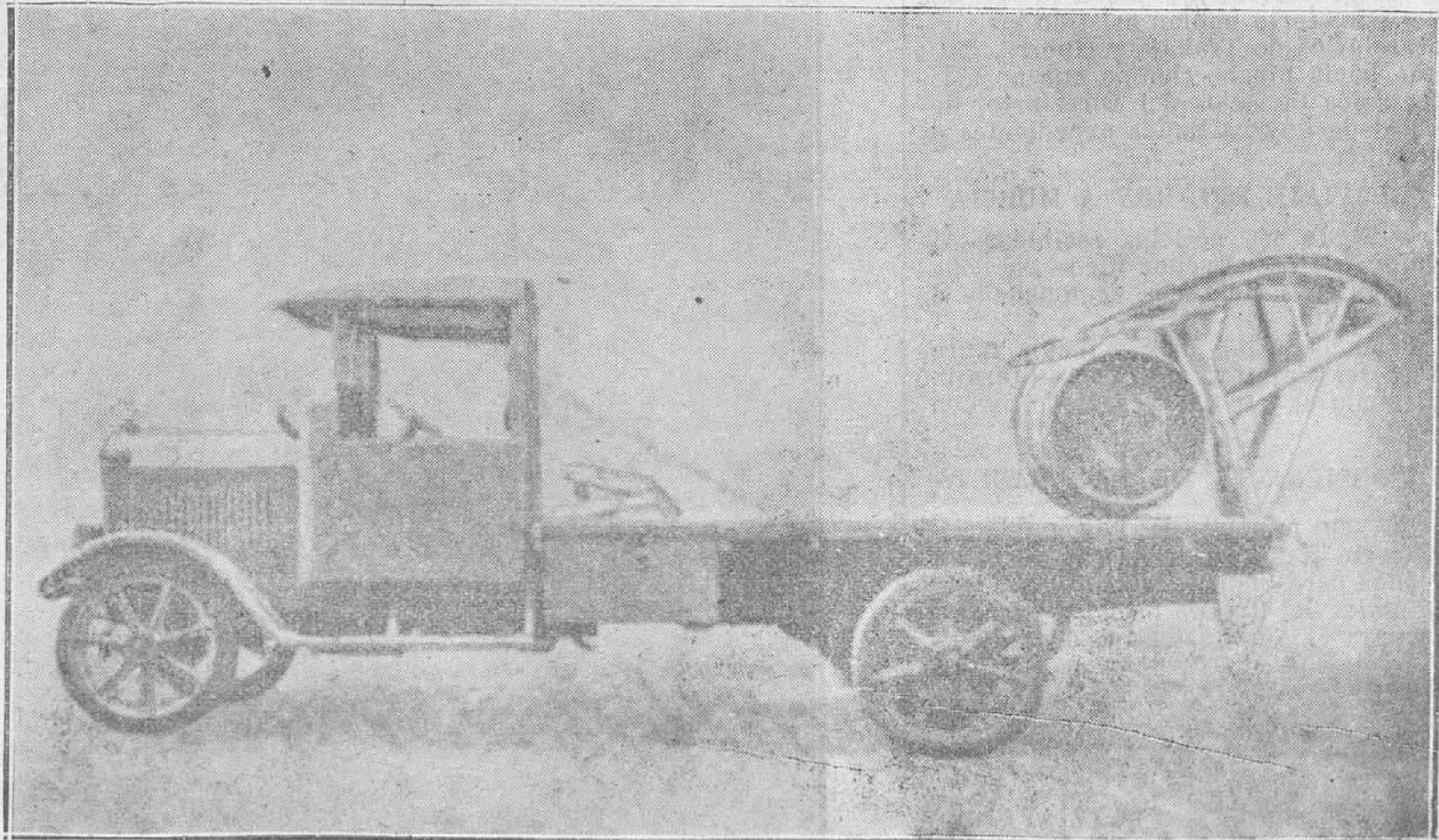
CUANDO LA OPERACION HA TERMINADO, EL BASCULADOR OCUPA PO CO SITIO.—La descarga del tonel se efectúa luego realizando las mismas operaciones en orden inverso.
