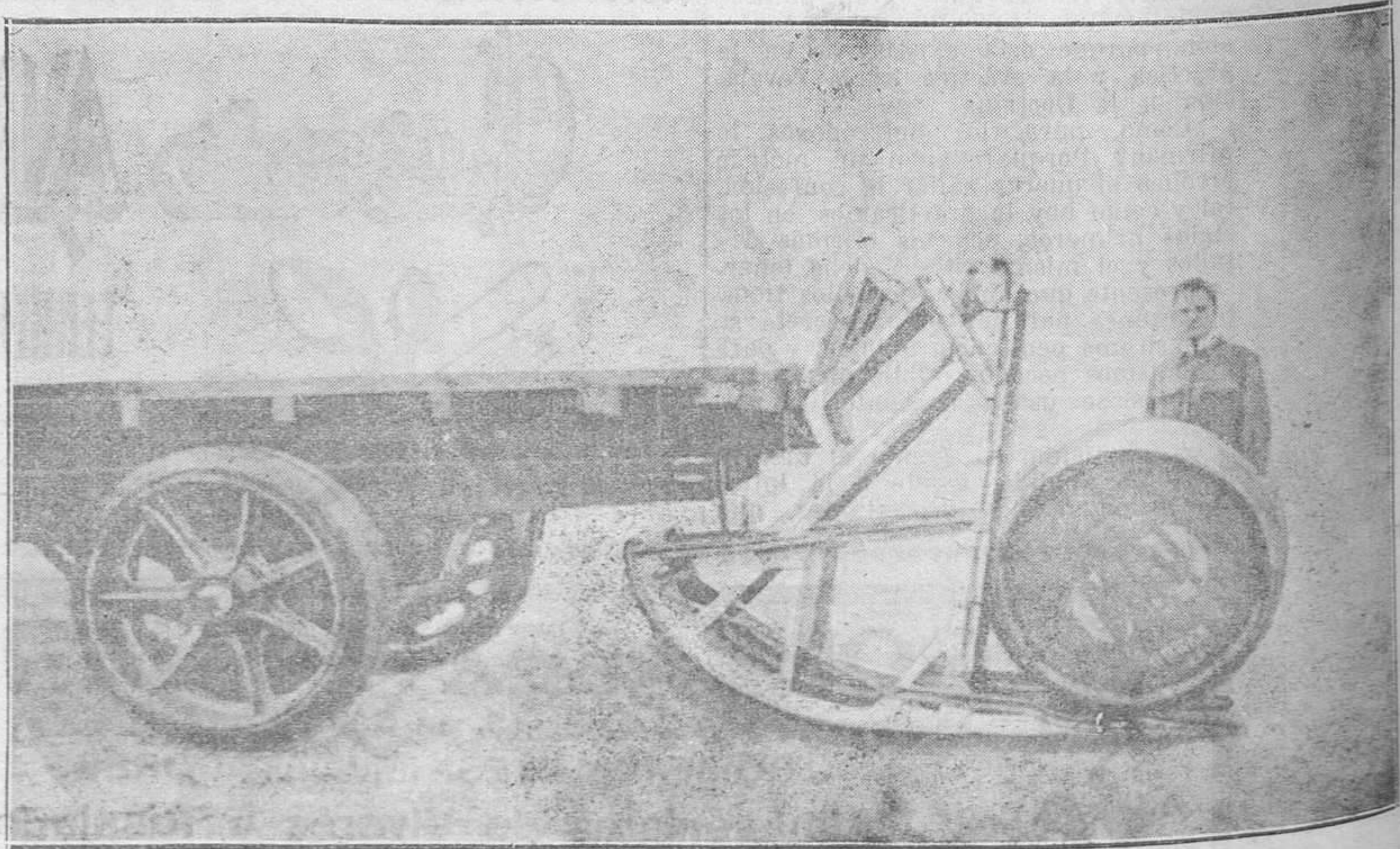
PRIMERA FASE DE LA CARGA DE UN TONEL EN UN CAMION.--Estando abatido el aparato sobre el suelo, se rueda el tonel hasta que repose sobre los montantes del basculador automático.
