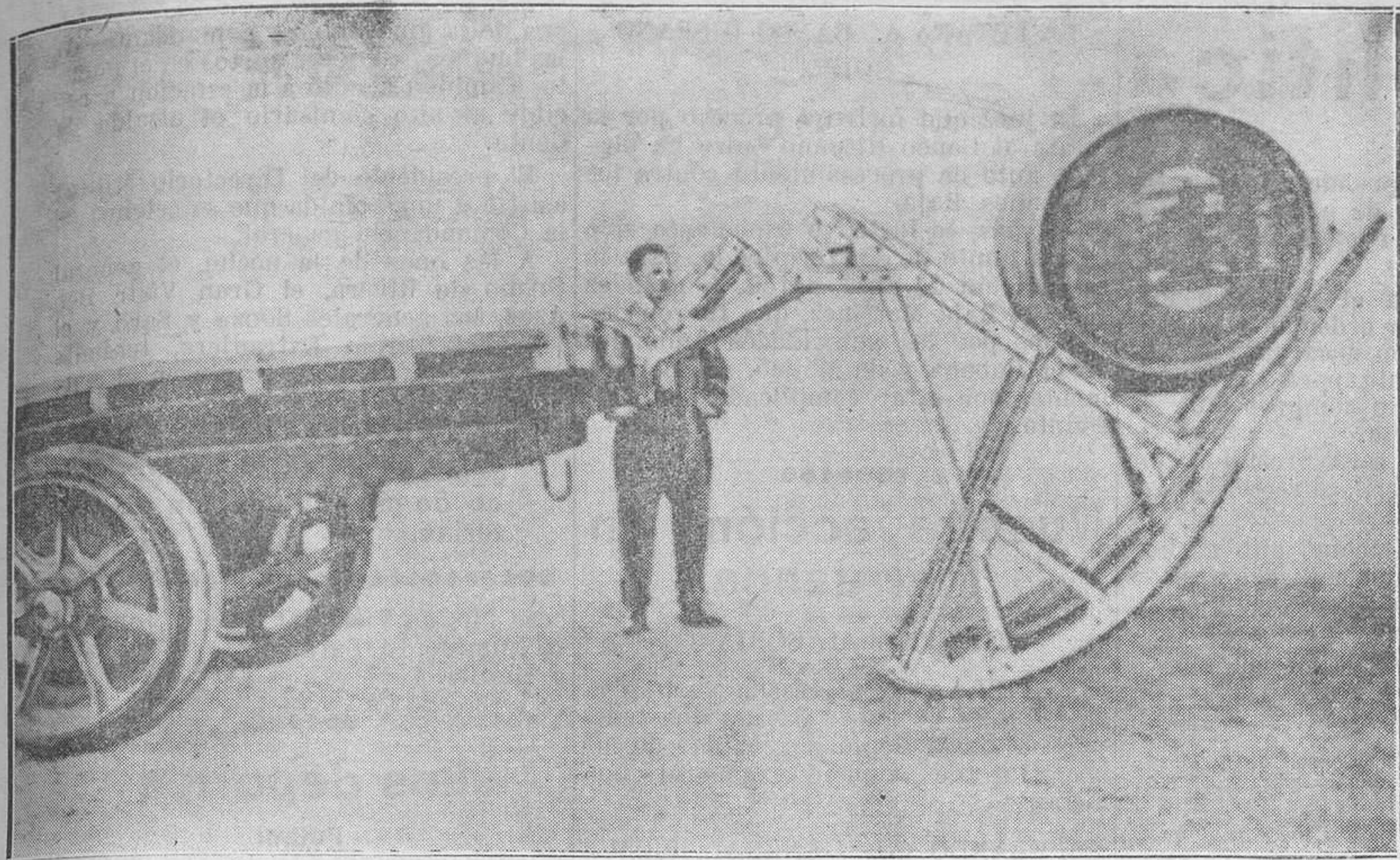
CUANDO EL CAMION AVANZA, EL TONEL SE ELEVA AUTOMATICAMENTE.—El aparato bascula en torno de su eje y eleva el tonel. Cuando este se encuentra a la altura deseada se le hace rodar.
