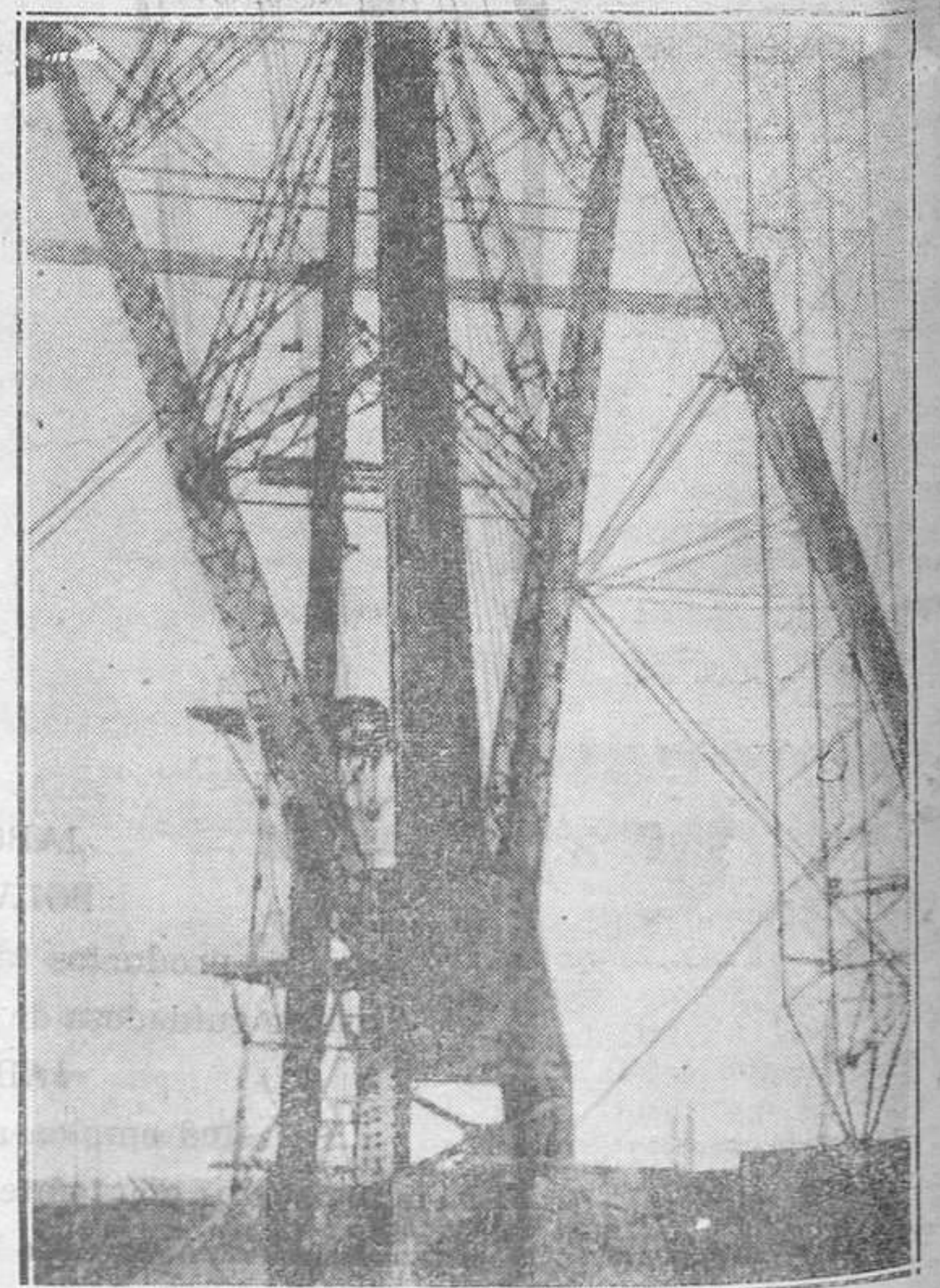
KOENIGSWUSTERHAUSEN.--La base metálica de un pilar de la estación de T. S. H. Mide de alto el pilar 225 metros y soportará la antena de la estación radiotelefónica. Según los alemanes esta estación será la más potente del mundo.
