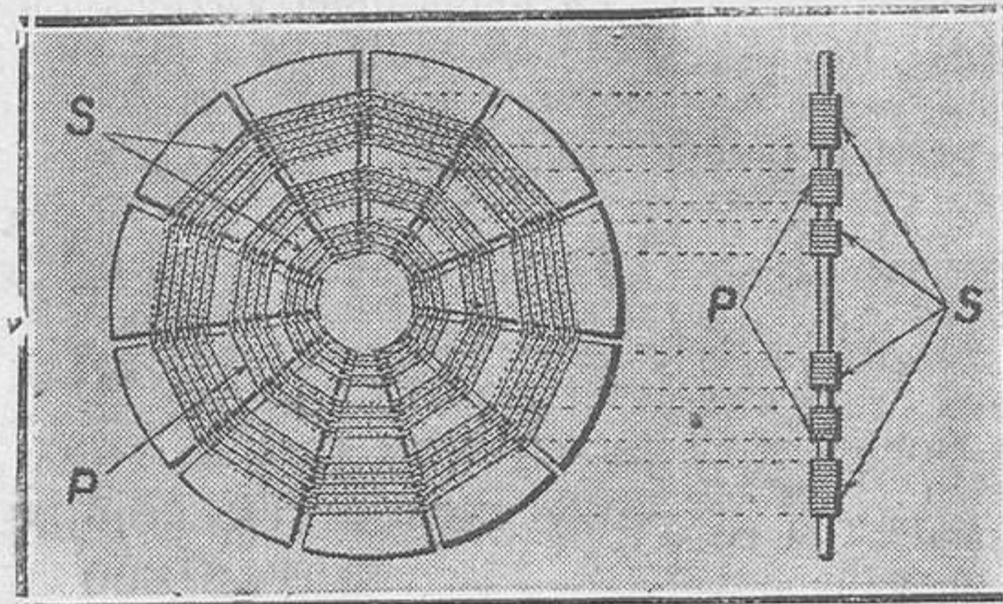
Fig. 2.--Bobina de acoplamiento del circuito de la antena con el circuito oscilante primario.
