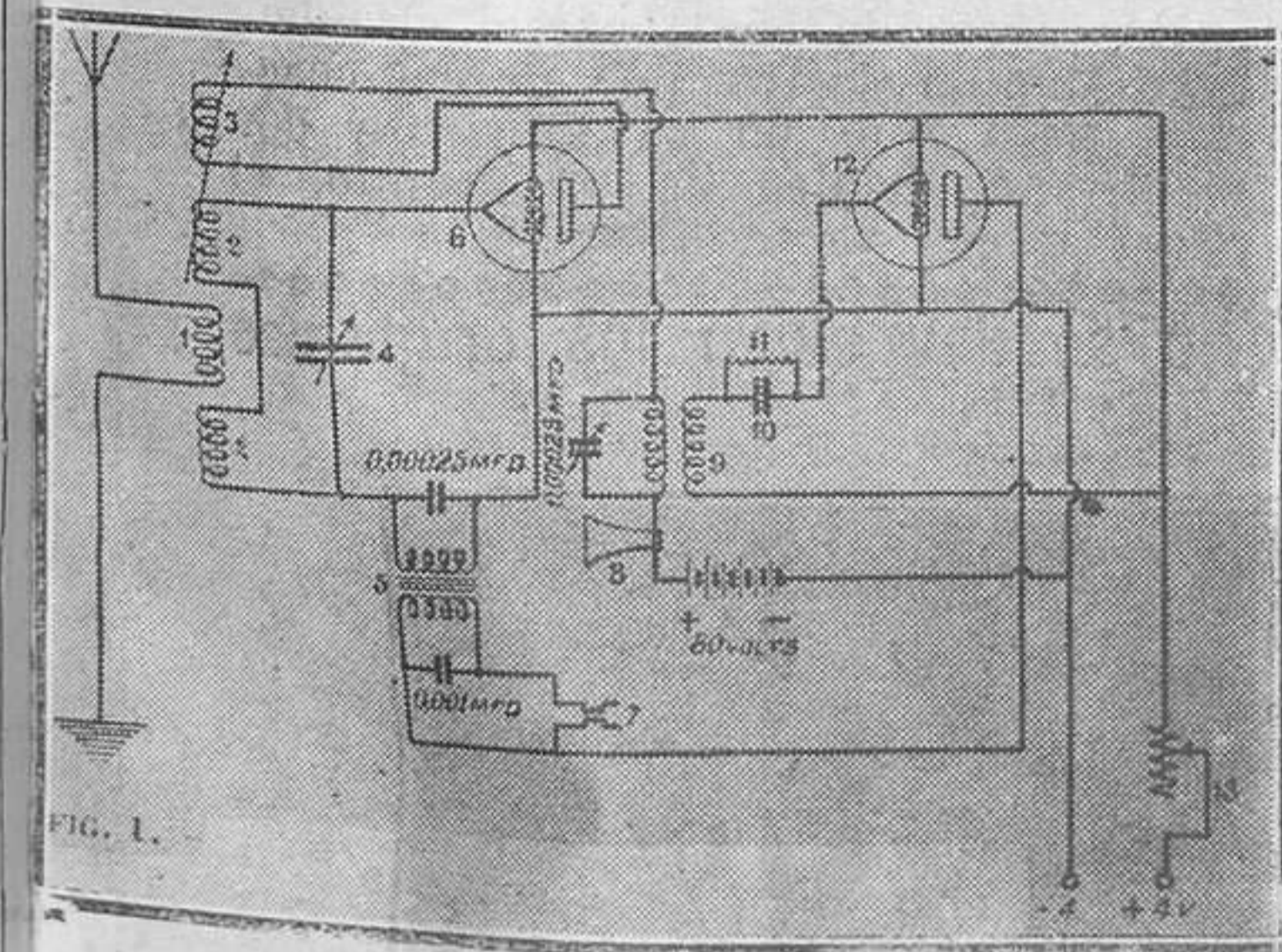
Figura 1.--Esquema general del montaje "Reflex".-- 1, bobina del primario de 10 espiras; 2, bobina del secundario de 45 espiras; 3, bobina de reacción de 20 espiras; 4, capacidad variable de 0,5 por 1000; 5, transformador B. F., de relación 1 por 10; 6, primera lámpara; 7, jack que permite recibir sin utilizar el efecto "reflex"; 8, alta voz; 9, transformador H. F., de hierro; 10, capacidad de 0,2 por 1000; 11, resistencia de 5 megohms; 12, segunda lámpara; 13, restato de 2 ohms.
