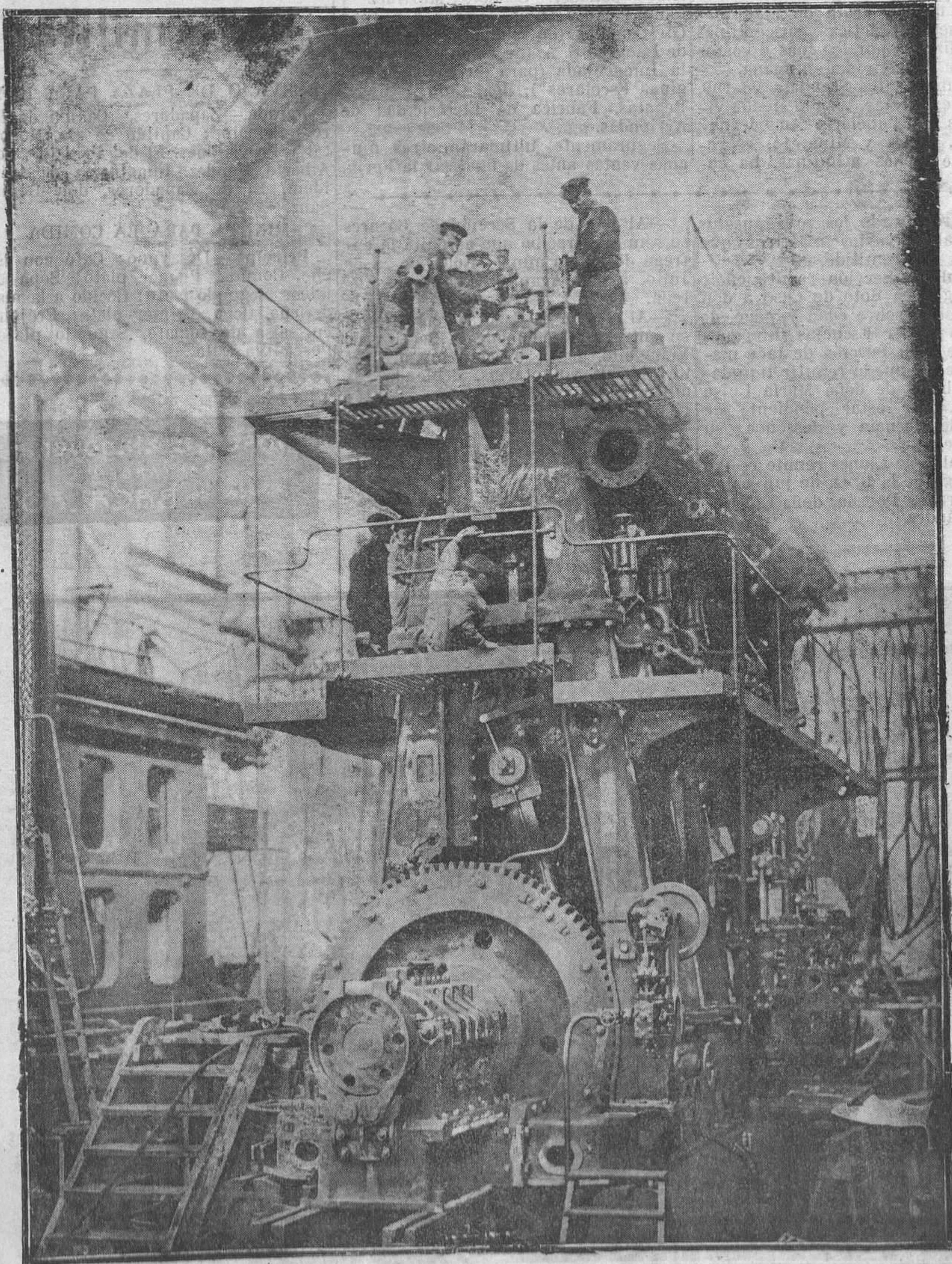
KIEL (ALEMANIA).—El motor Diesel el mayor del mundo que se está construyendo por los alemanes para Inglaterra a cuenta de reparaciones de guerra. (Foto Vidal)
