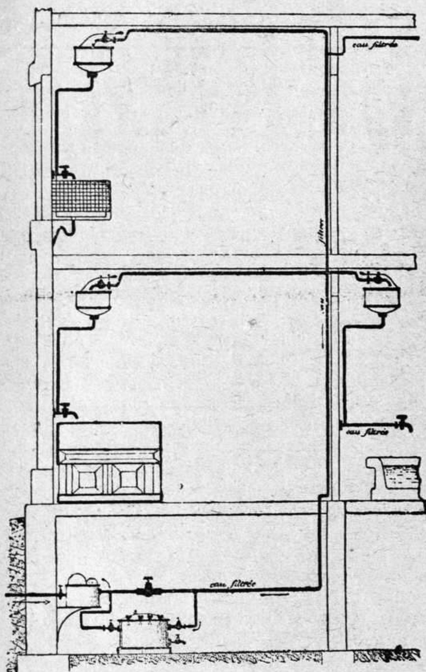
Instalación de una batería de filtros surtiendo de agua, los diferentes pisos de una casa.
