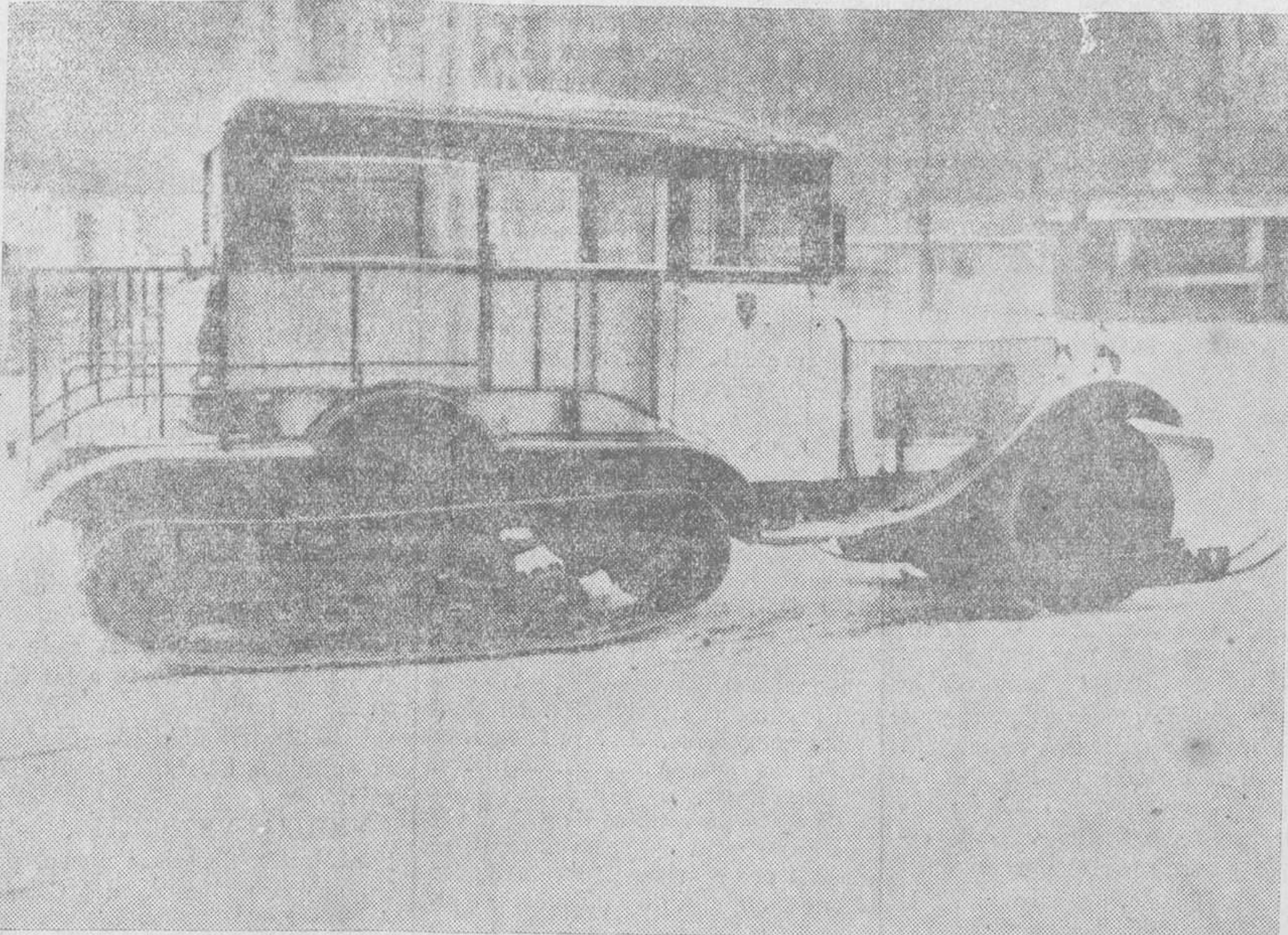
La Administración de los Correos de Austria acaba de poner al servicio un nuevo modelo de autobús destinado al transporte de los viajeros por los caminos cubiertos de nieve. La característica de estos vehículos consiste en que, en vez de las ruedas traseras, hay un sistema de «corugas», mientras que las delanteras llevan un par de skis, en todo lo cual son imposibles los resbalones. La fotografía muestra el nuevo autobús de la Administración de Correos de Austria.
