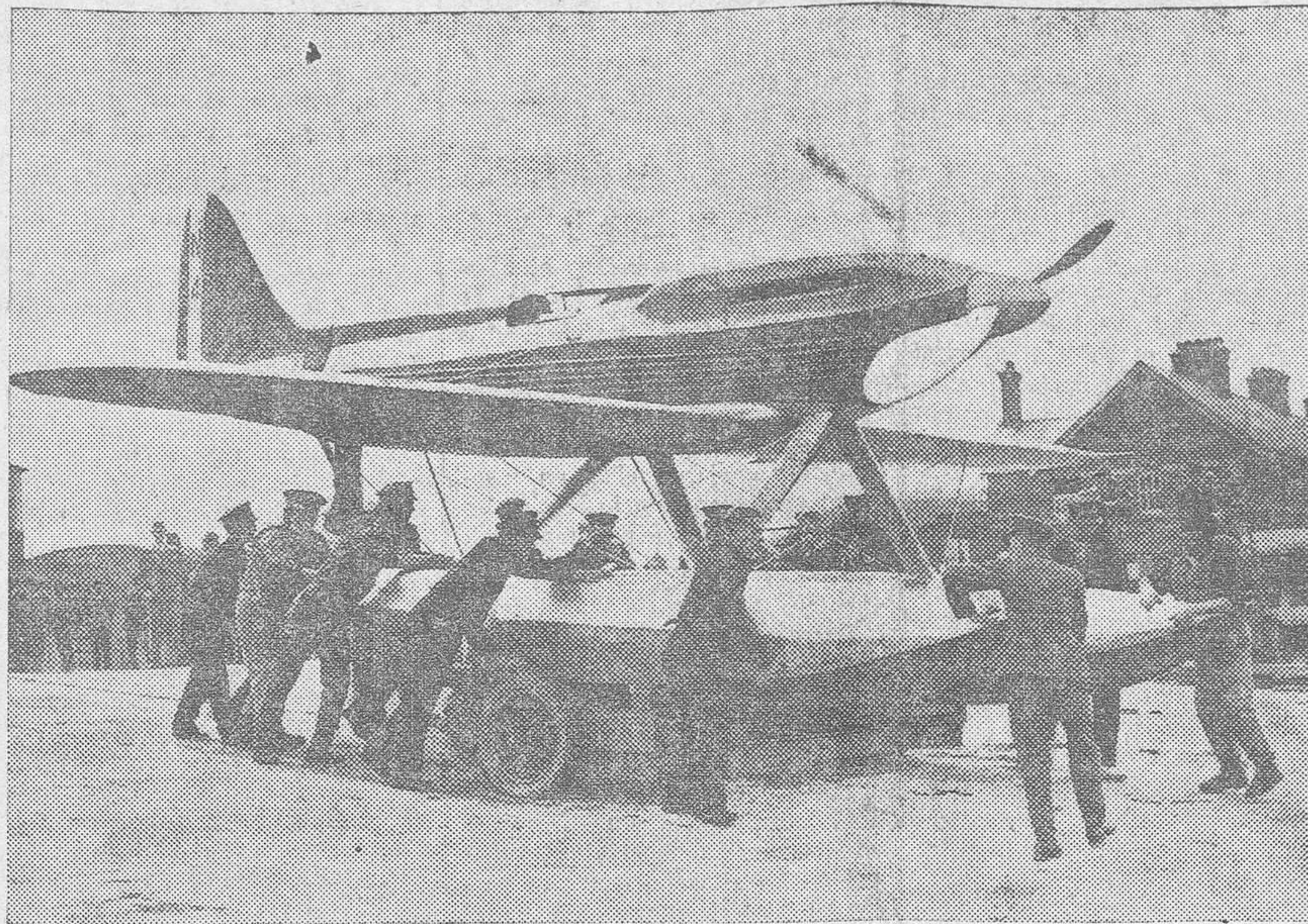
Amarado para pruebas en Calshot hay uno de los aparatos supermarinos «Rolls-Royce S. 6» que representará a la Gran Bretaña en la carrera de la copa Schneider en el Gólcot en septiembre. Se espera que alcance una velocidad de unas 300 millas por hora
