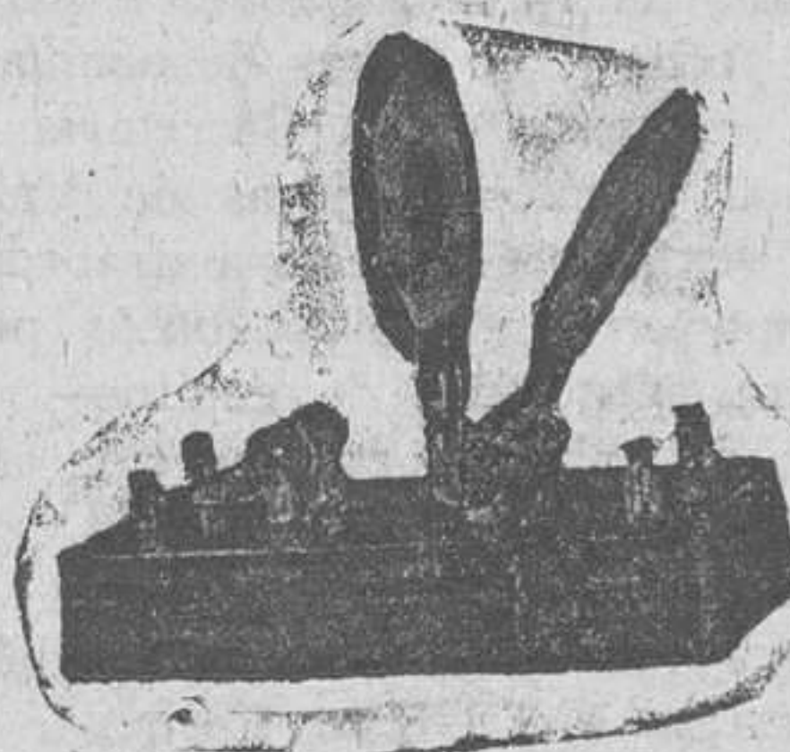
Receptor de galena. Tipo núm. 4.805. Precio: 14 pesetas.
