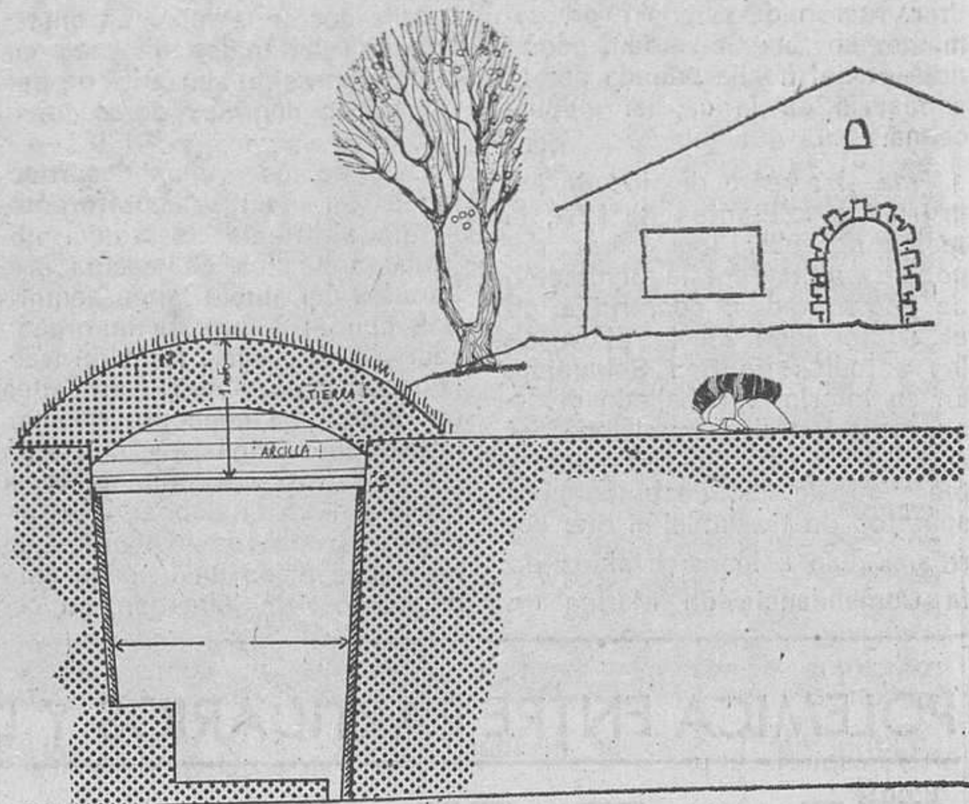
Esquema de un refugio particular, construido con materiales al alcance de la mano. Se cava un hoyo y se cubre con vigas de madera y un metro de tierra y arcilla. Las paredes interiores se revisten con cañas bien sujetas.
