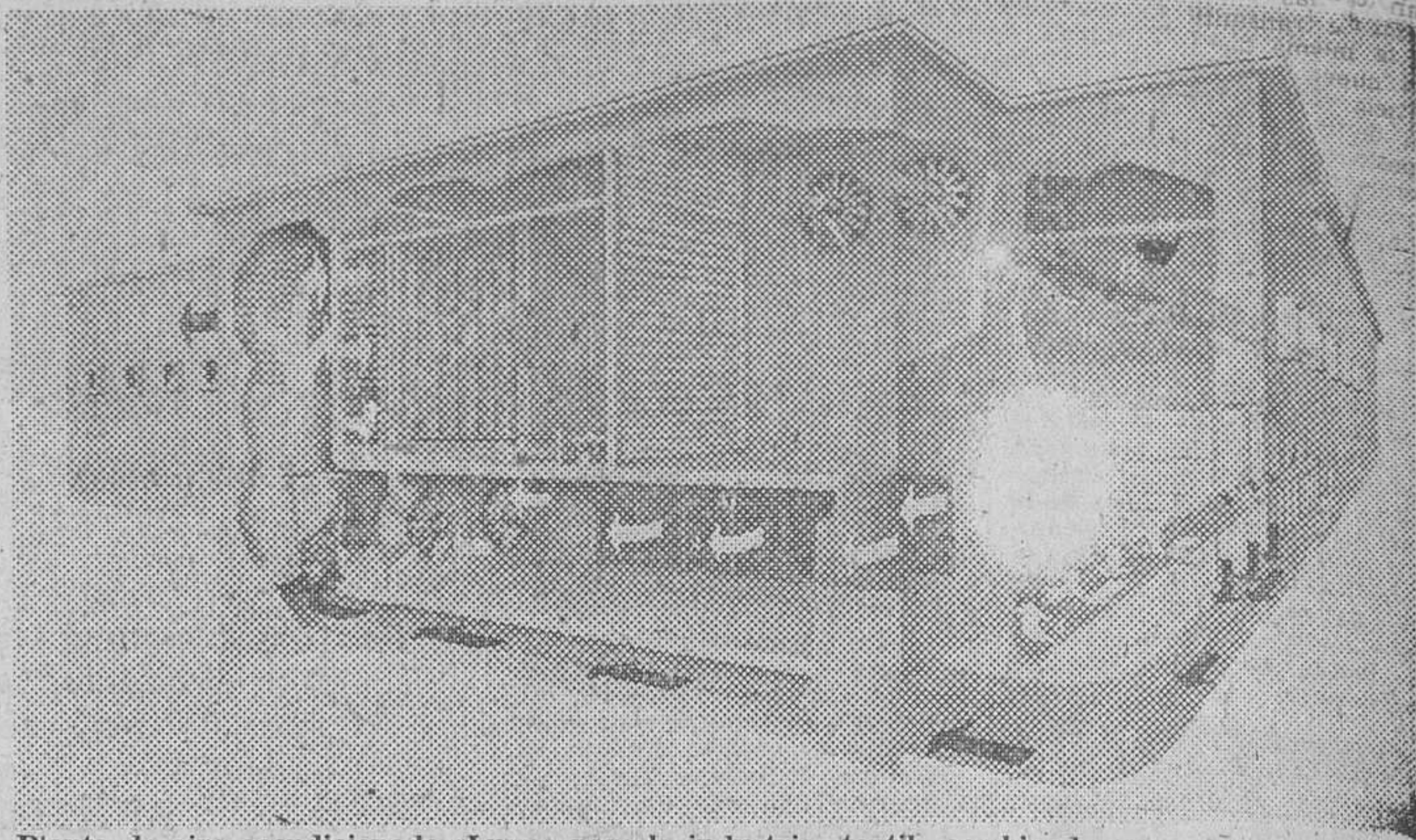
Planta de aire acondicionado «Luwa» para la industria textil, combinada con equipo central de succión «Pneumafil»
