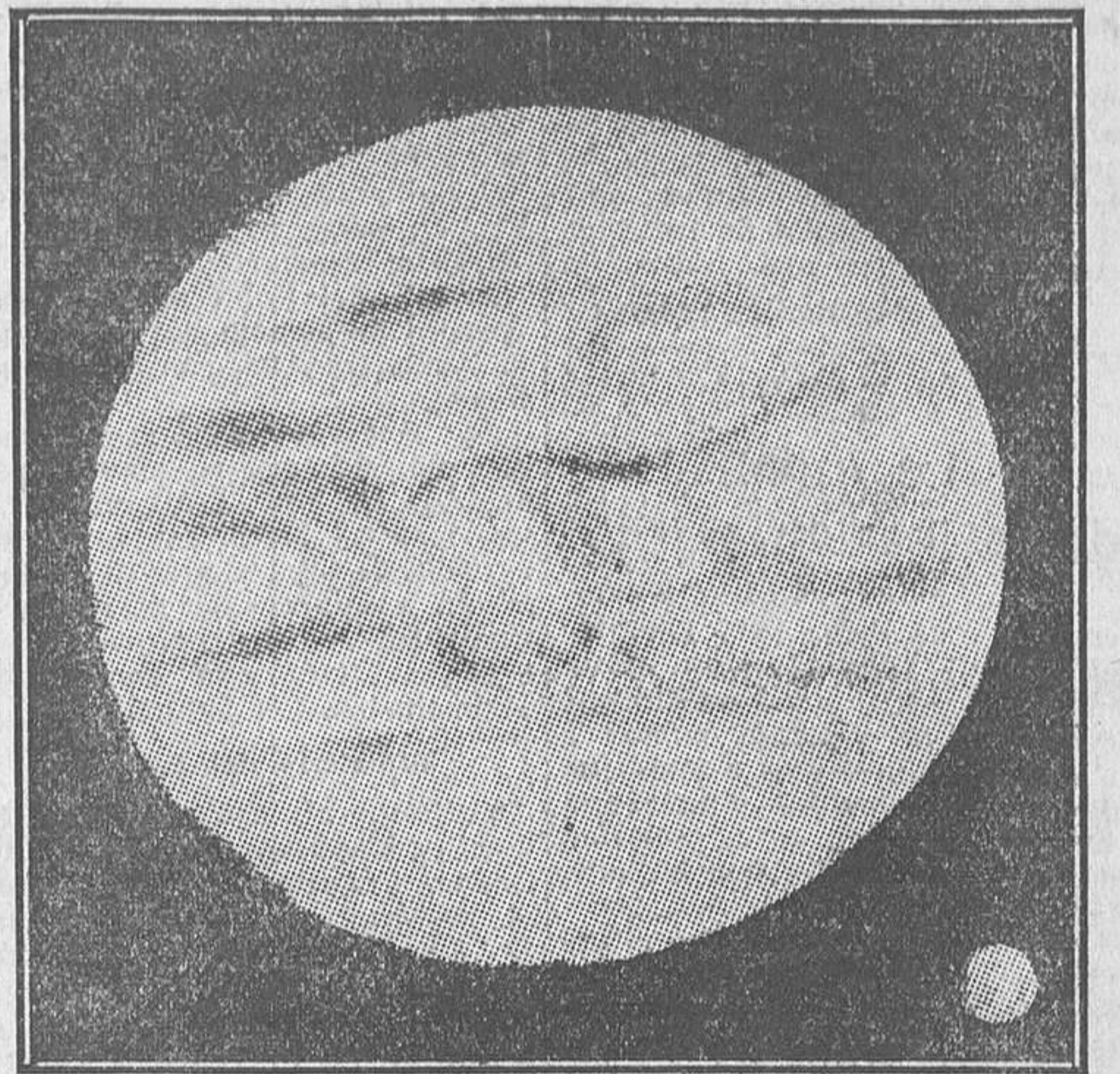
Aspecto del planeta Júpiter en el campo de un potente anteojo. En un ángulo se ve la Tierra dibujada a escala
