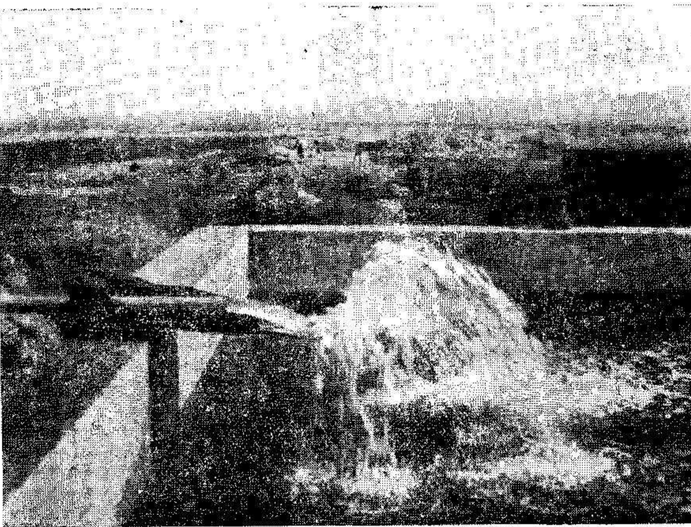
Instalación de riego (60.000 litros hora) efectuada por la Casa Tortosa & López Avalos, en la finca de Ismael Sadre en la kabila de Barraca (Nador) (Foto Tortosa)
