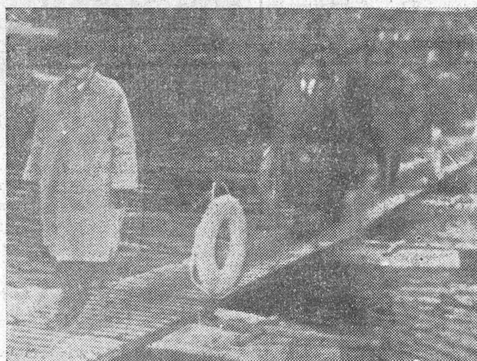
Fuerzas de Ingenieros de Salamanca, tendieron en poco más de veinte minutos dos puentes sobre flotadores para facilitar el paso sobre el Tera y comunicar la carretera con Ribadelago. Las "fotos" nos muestran a los soldados en pleno trabajo, y una vez terminado, el paso de personas sobre uno de los puentes. En una de estas "fotos", el señor Ministro de Obras Públicas utiliza el nuevo y provisional paso.
