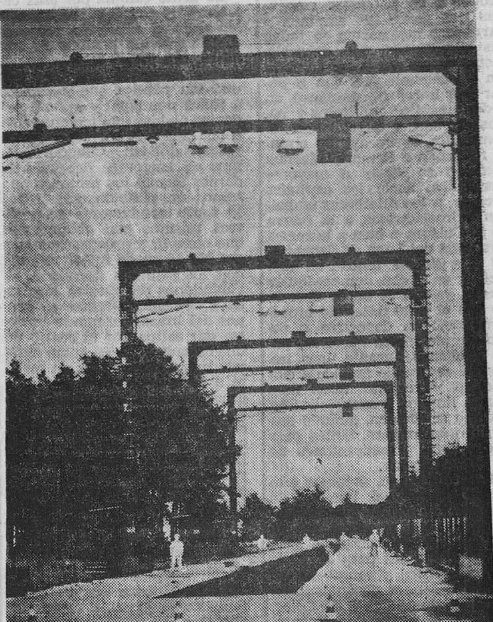
Imitaciones de hombres, tablas de contrastes y señales de tráfico, colocadas en la "Calle para ensayos de iluminación".
