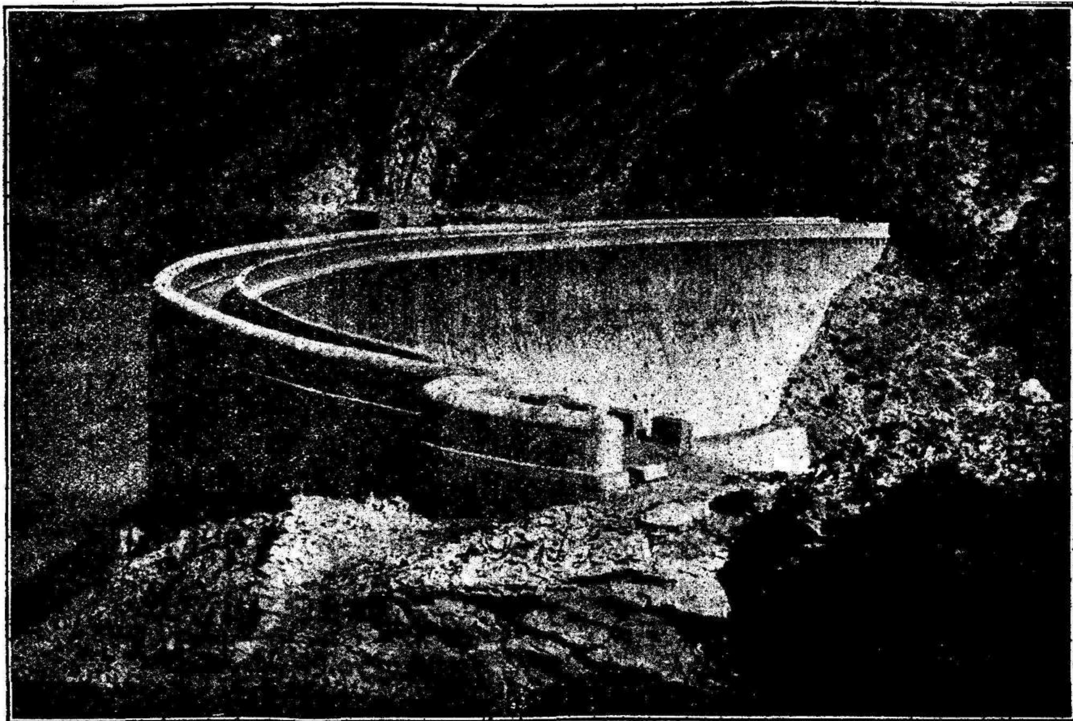
Regadío de Lorca.—Obras de embalse.—Presa del Pantano de Valdeinfierno en el río Luchena
