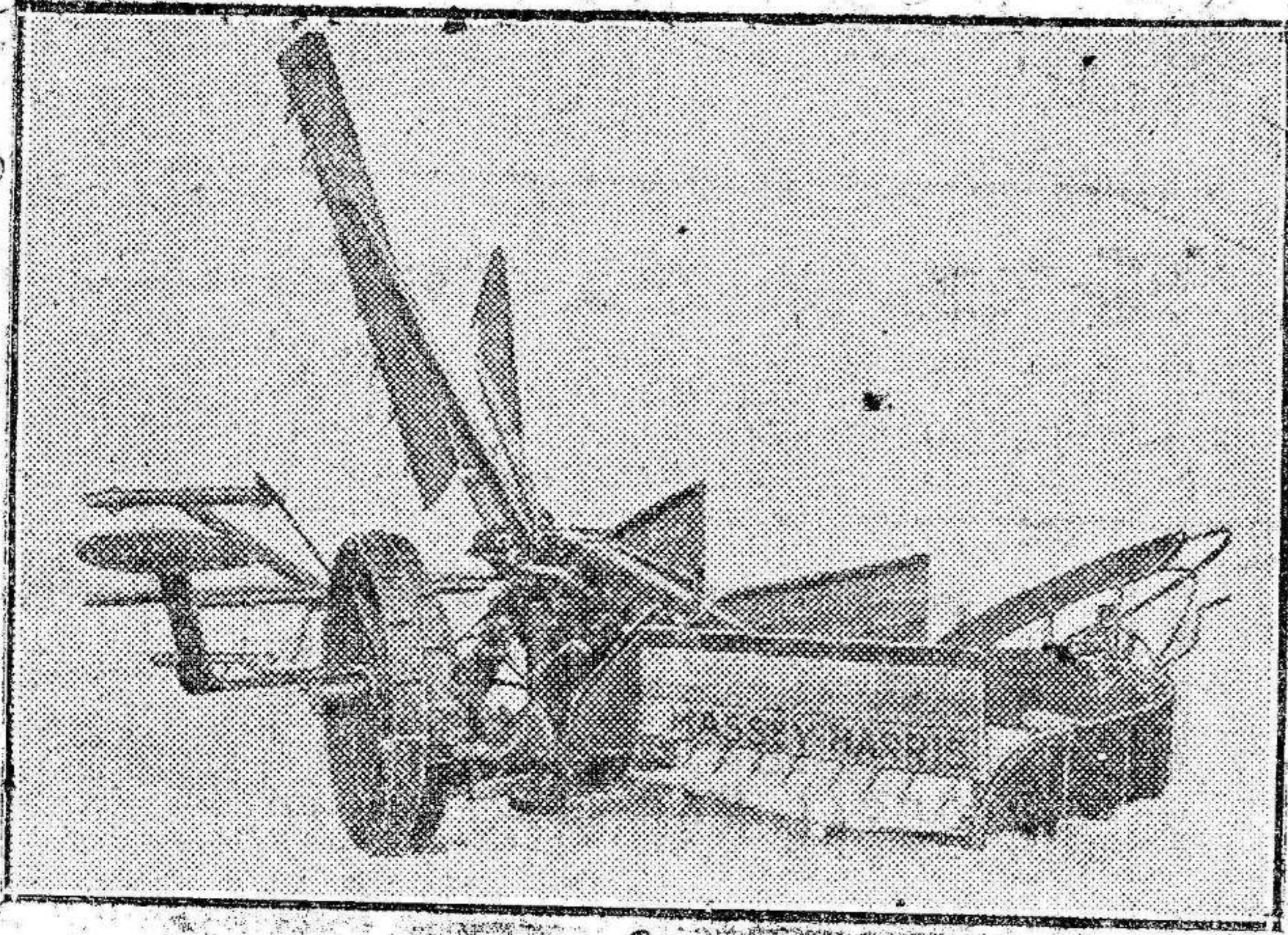
Gavilladora Massey-Harris número 2 DE ENGRANE LA SEGADORA IDEAL PARA ESPAÑA
