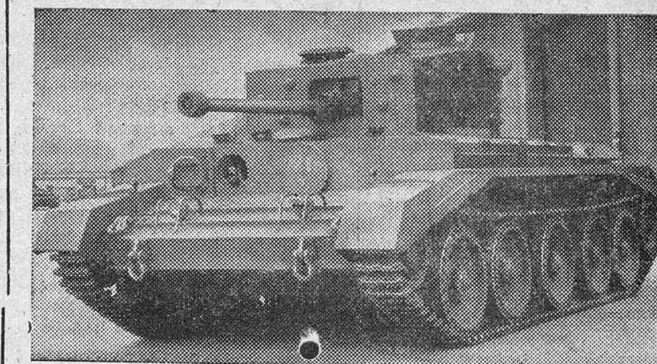
El novísimo tipo de tanque británico "Centaurio", usado con tanto éxito en las operaciones de Francia.
