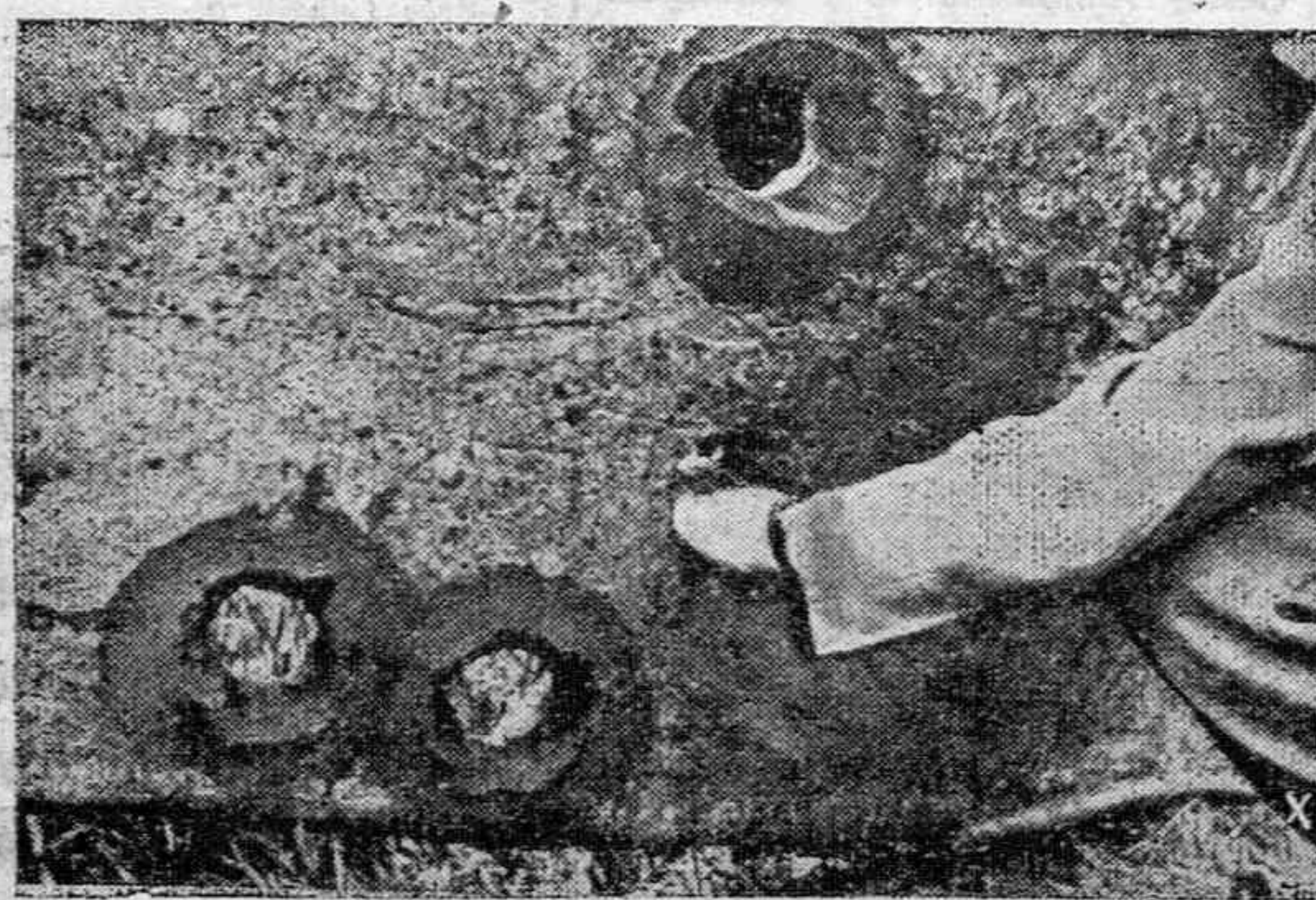
Esta fotografía nos muestra los efectos causados en la coraza de un tanque por un nuevo explosivo lanzado por el arma antitanque alemana.
