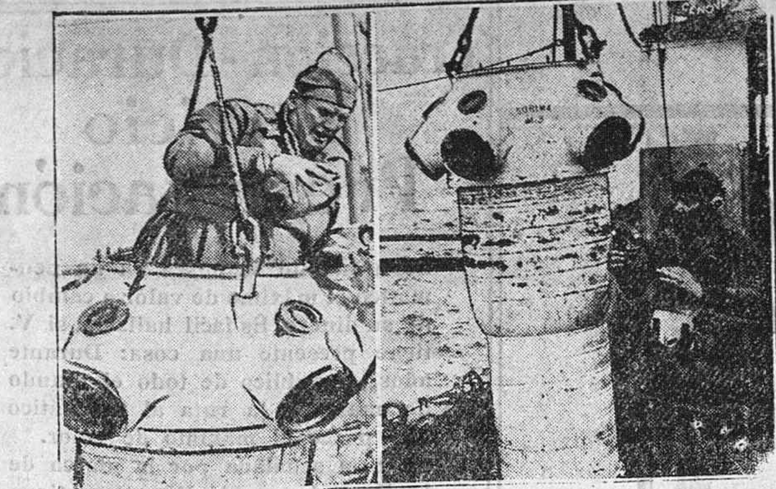
El paquebot «Egypto» fué echado a pique durante la guerra llevando en sus bodegas un importante cargamento de oro. Ahora una sociedad italiana, que ha conseguido poner varios barcos a flote, se ha hecho cargo de estos trabajos.—He aquí una escafandra usada por los buzos en el momento de empezar sus labores.
