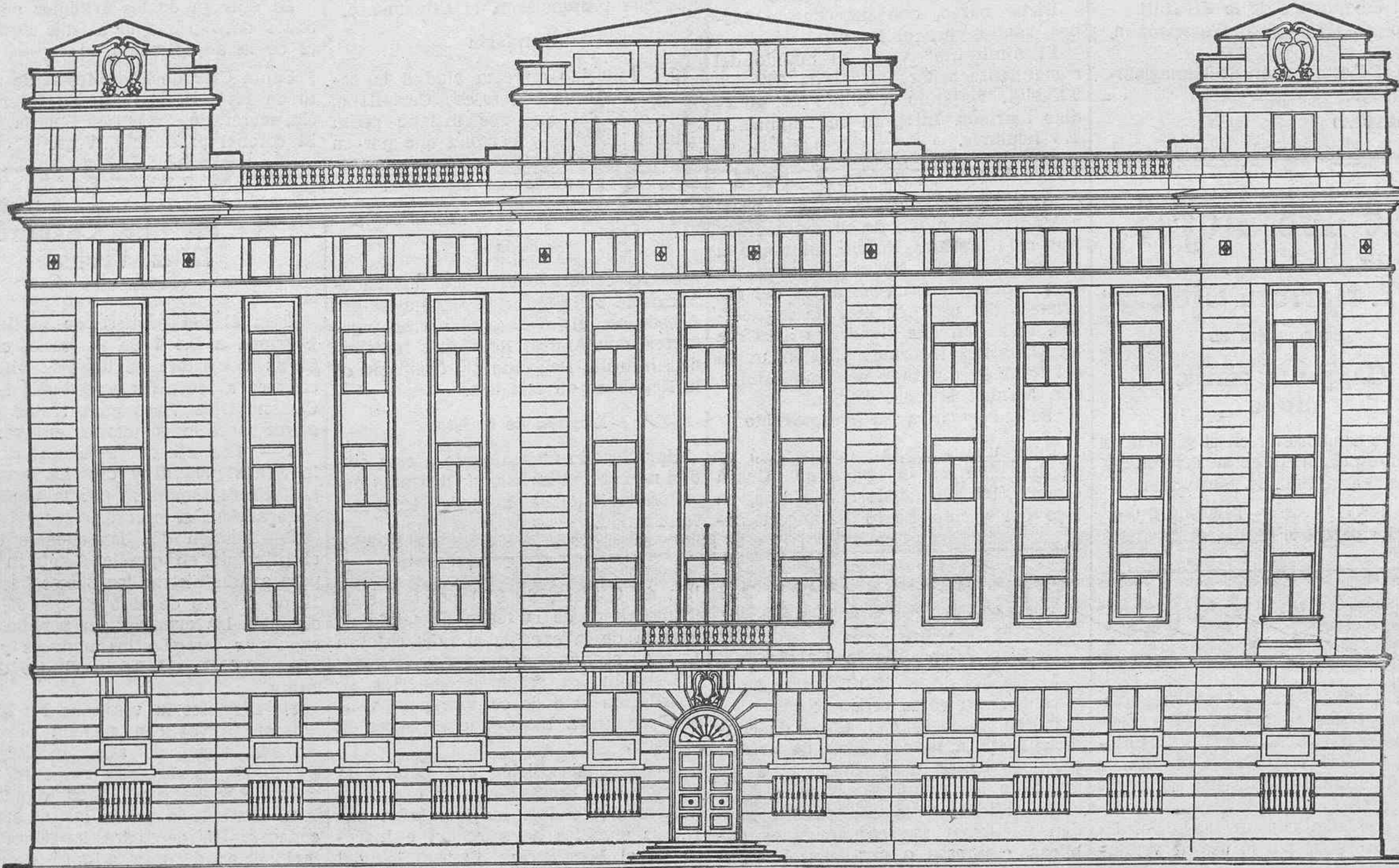
Plano de fachada del nuevo edificio para dependencias de Obras Públicas, proyectado por el Cabildo Insular acogidos a los beneficios de la Ley contra el Poro. Este magnífico proyecto, obra del arquitecto tinerfeño, don José Enrique Marrero, comprende: Una planta de semi-sótanos para garajes, laboratorios, etc.; un piso, el bajo, para la Junta de Obras del Puerto; otro para la Jefatura de Obras Públicas; otro para la Junta Administrativa de Obras Públicas; otro para la Junta del Grupo de Puertos de La Palma y la superior dedicada a vivienda de jefes y conserjes de las distintas dependencias. La fachada central de este edificio dará frente a la explanada del muelle y las laterales a la calle central y a la prolongación de la del Sol.
