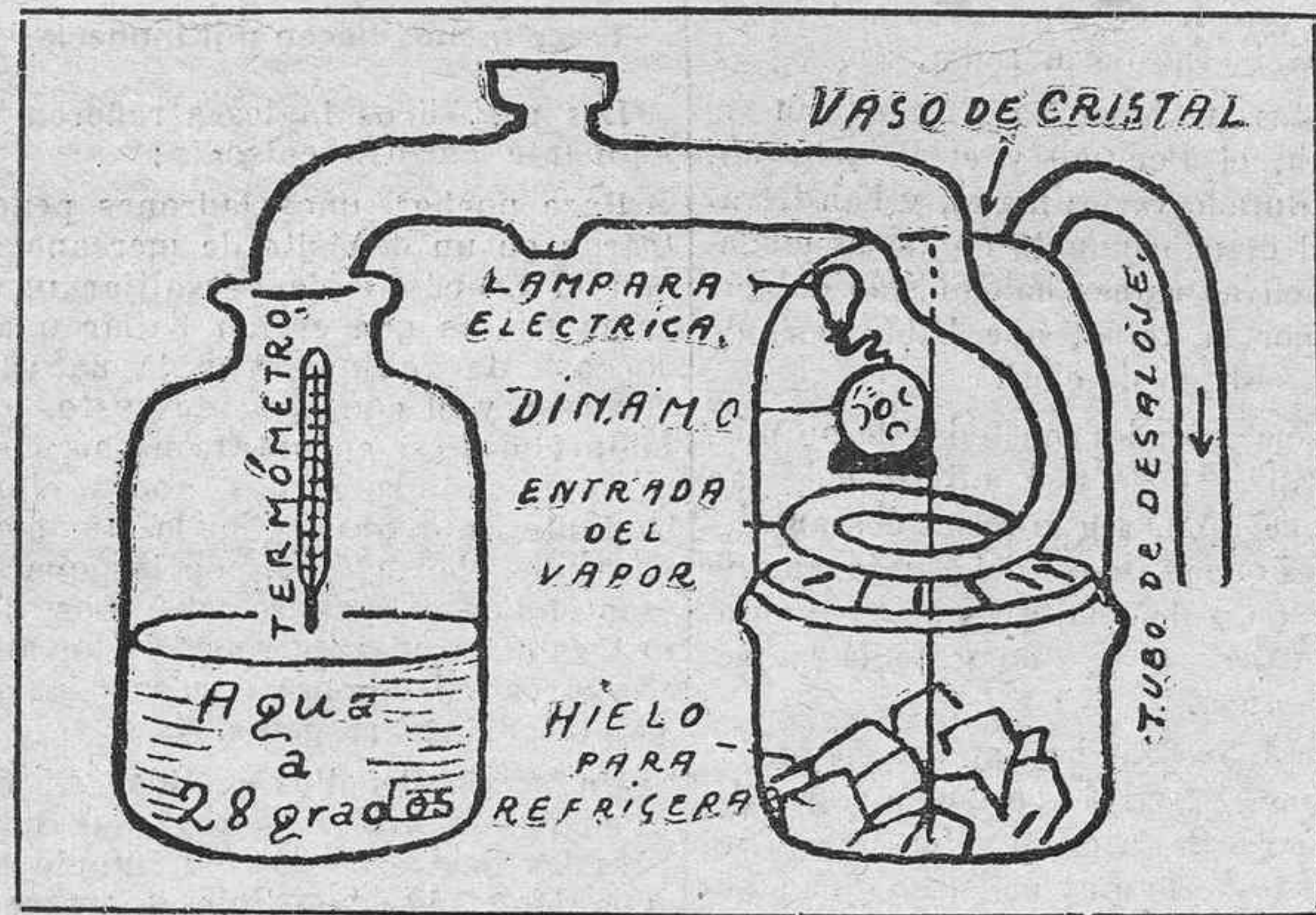
EL CURIOSO EXPERIMENTO DE M. CLAUDE PARA UTILIZAR LA ENERGIA DE LOS MARES.—El eminente sabio con el nuevo aparato que ha dado a conocer en la Academia de Ciencias de París, para utilizar la energía de los mares como fuerza motriz.—Esquema del curioso aparato y del funcionamiento del mismo
