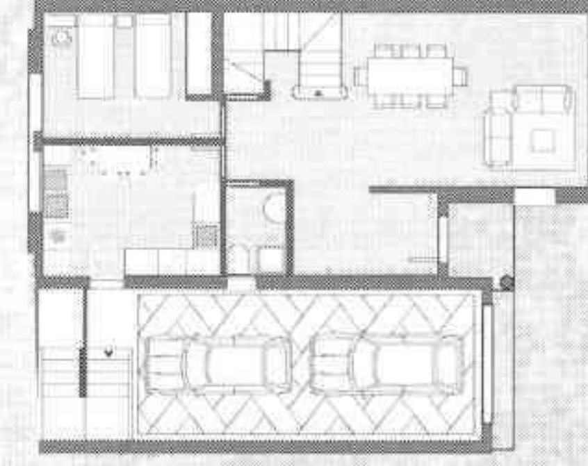
Modelo Herrera Individual, 4 dormitorios Sup. construida 232,82 m 2
