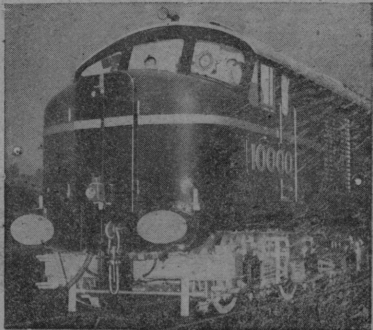
La nueva locomotora L. M. S., número 10.000, es impulsada por un motor Diesel English Electric de 1.600 HP. y 16 cilindros, y está destinada a trabajar independientemente o acoplada a una segunda unidad en construcción para formar una locomotora de 3.200 HP., capaz de arrastrar el expreso más pesado y de alcanzar una velocidad máxima de 160 kilómetros por hora. El empleo de estas locomotoras permitirá un apreciable ahorro de carbón. (Calpe).
