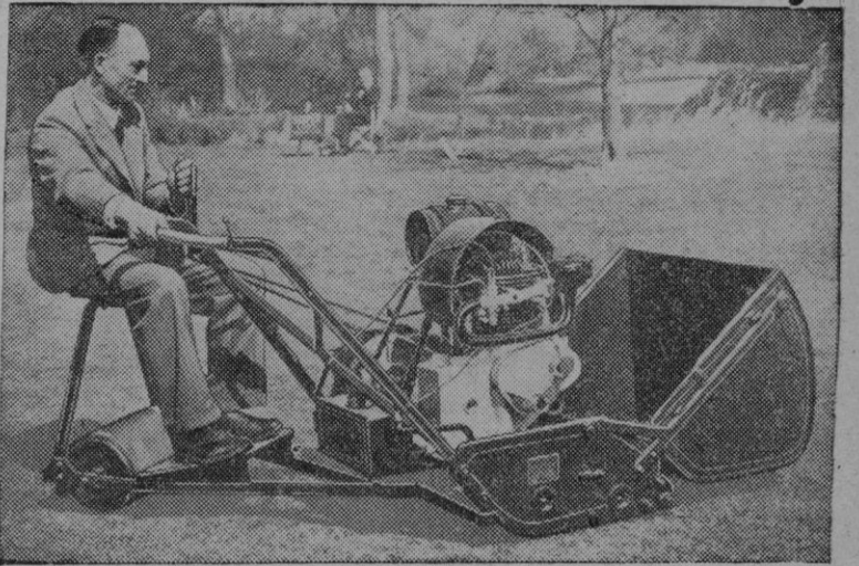
Un invento más para la horticultura. — Una segadora, accionada por un motor de 4'5 a 7 HP., con asiento, cuya base actúa de ro-Real Sociedad de Horticulturadillo adicional, presentada en la británica
