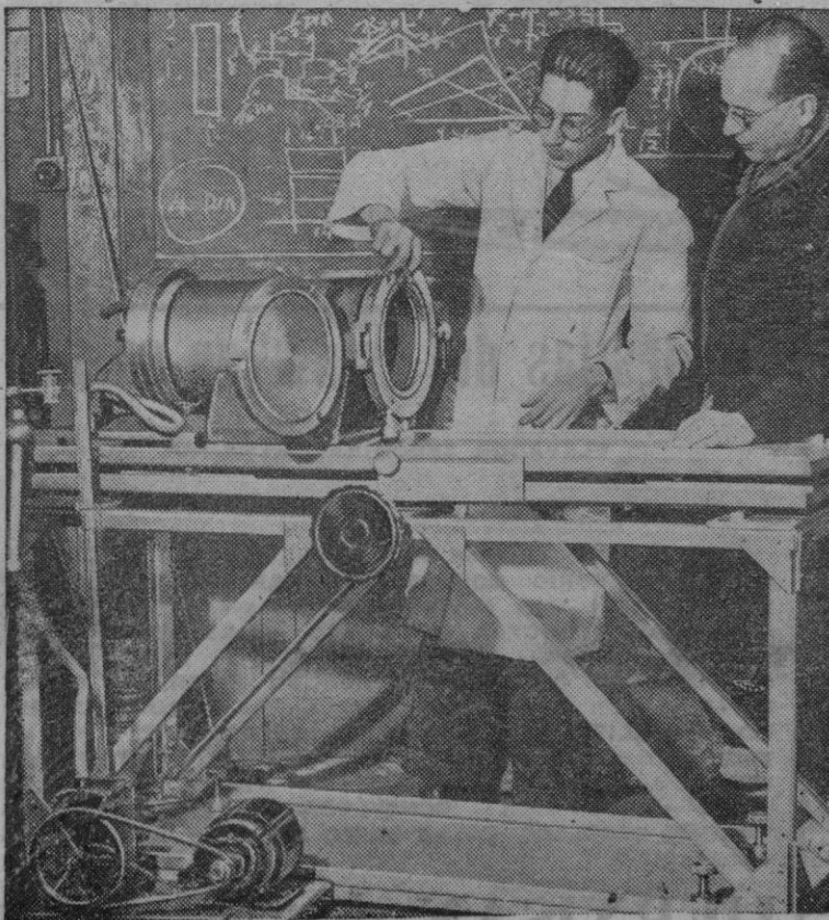
El Dr. Bannister durante una demostración en la Universidad de Bristol, con la máquina de dispersión para fotografiar las huellas de los átomos
