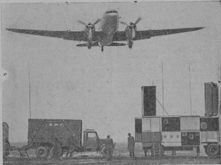
La mayor seguridad en los vuelos cuando el tiempo es adverso se debe al aparato G.C.A. (Control de llegada desde Tierra) instalado recientemente en el aeropuerto de Londres. Al contrario de lo que ocurre con la mayor parte de los sistemas radar, T.G.C.A. no exige que el avión esté dotado de una instalación especial de radio, aparte de los receptores de comunicación normales.
