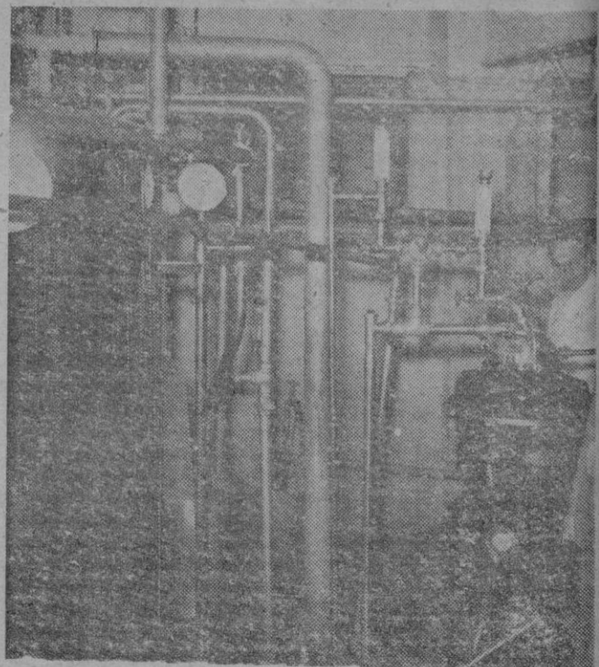
El pasturizador, uno de los aparatos más importantes que funcionan en la instalación modelo de CENTRAL LECHERA.
