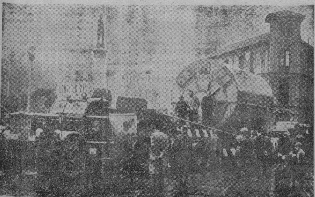
La Polguerra. — Para el transporte del "estator" de 75 toneladas destinado a la central eléctrica de la Polguerra, se precisó un camión especial de 28 ruedas, que media 22 metros de longitud, y transportaba, además, un transformador de otras 75 toneladas.
